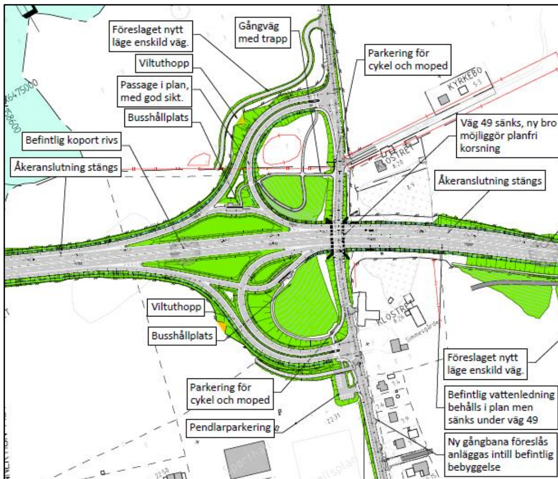
Bild 4.2.3. Utformning av trafikplats Varnhem med bland annat busskörfält, gång- och cykelvägar och pendlarparkering. Norr är rakt upp i bilden.
