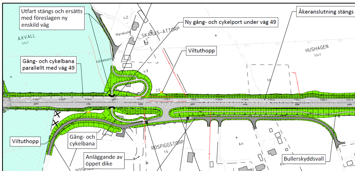
Bild 4.2.5. Den nya korsningen mellan den tillkommande enskilda vägen och väg 49 samt ny gång- och cykelport "Rospiggstorp". Norr är rakt upp i bilden.
