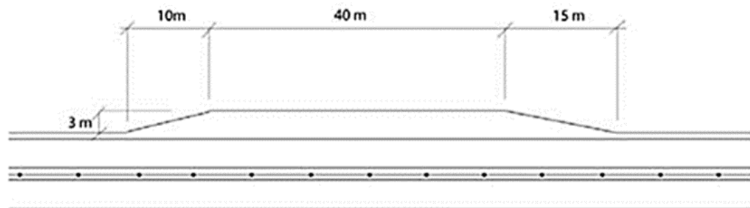
Bild 4.2.2-2. Utformning av nöduppställningsplats (benämns ficka i tabellen nedan). De ska rymma en lastbil med släp samt en bärgare.
