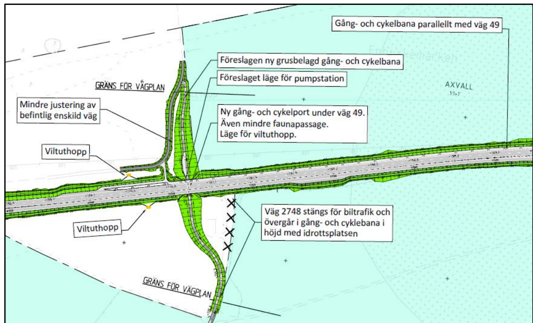
Bild 4.2.4-2. Ny gång- och cykelport under väg 49 vid Hedvägen (väg 2748) samt ny gång- och cykelväg på den norra sidan, parallellt med väg 49 över Axevalla hed. Norr är rakt upp i bilden.
