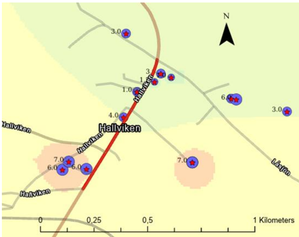
Figur 4.6:3 - Utdrag från SGU:s jorrdjupsmodell med Jorrdjupsobservationer från brunnnsdataarkivet. Röda färgen indikerar djup på 5–10 m, gul indikerar 3–5 m och det ljusgröna 1–3 m.
