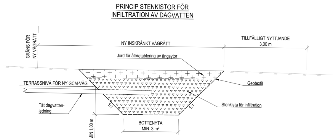
Figur 5.2:1 – Principskiss över stenkistor för infiltration av dagvatten.
