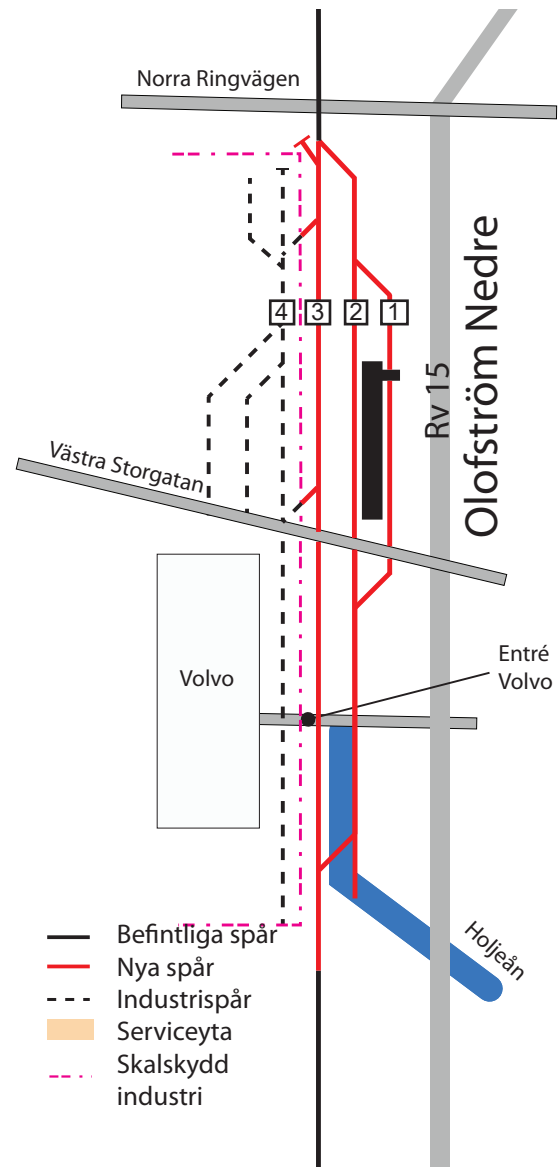
Figur 4.4 Schematisk skiss av Olofström nedre.
