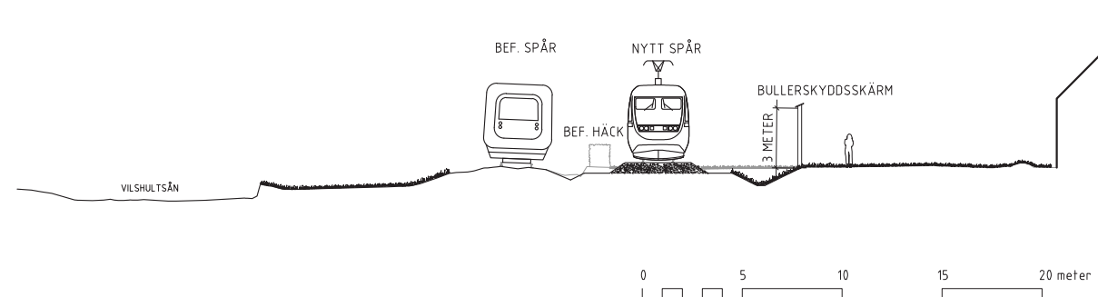
Figur 5.3 Typsektion som visar befintlig järnväg, det nya angöringsspåret samt bullerskyddsskärm vid Norra Holje.
