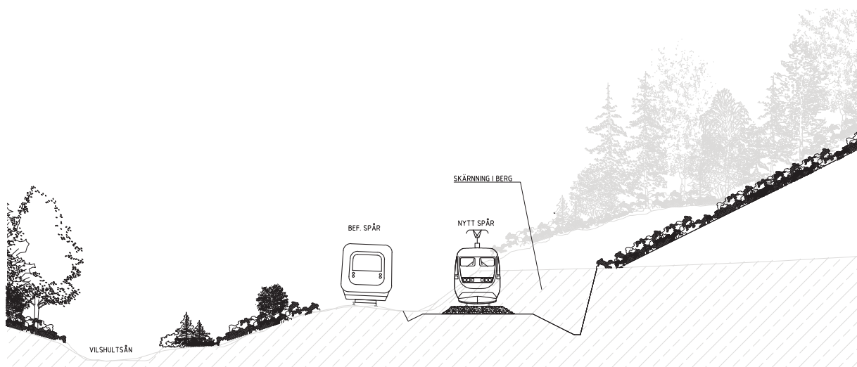
Figur 5.1 Typsektion som visar angöringsspårets påverkan på landskapet där det går i bergskärning.
