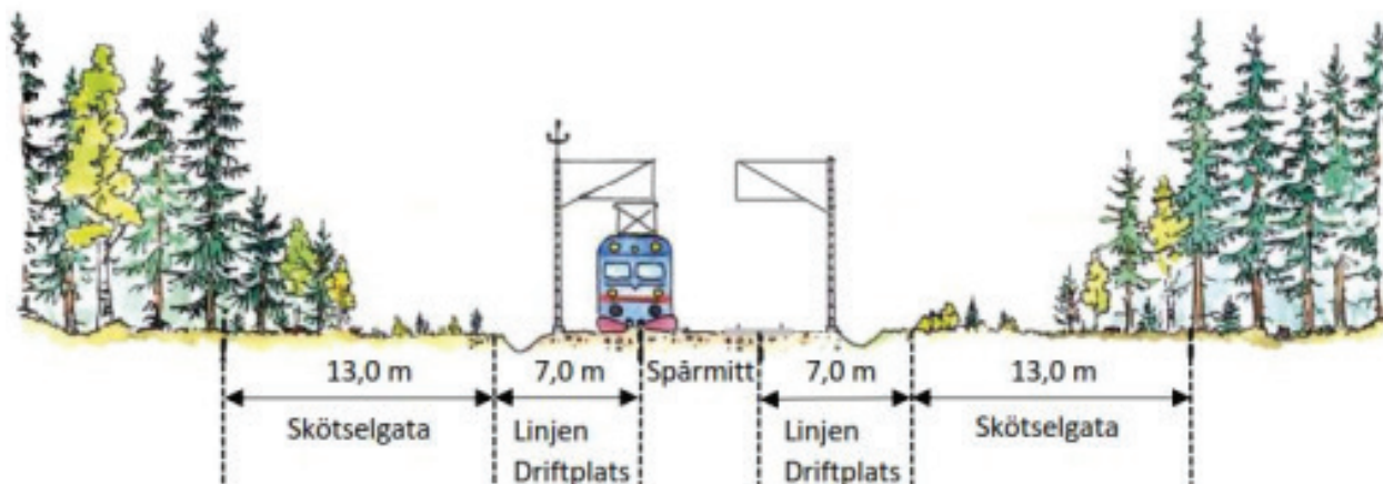
Figur 4.8 Princip för trädsäkring.
