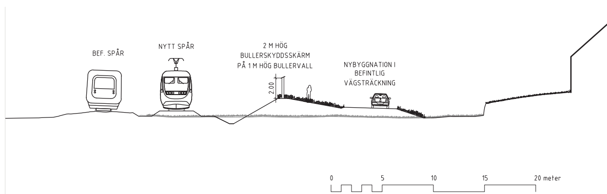
Figur 5.2 Typsektion som visar befintlig järnväg, det nya angöringsspåret och den kombinerade bullerskyddsvallen och skärmen vid Norra Holje.
