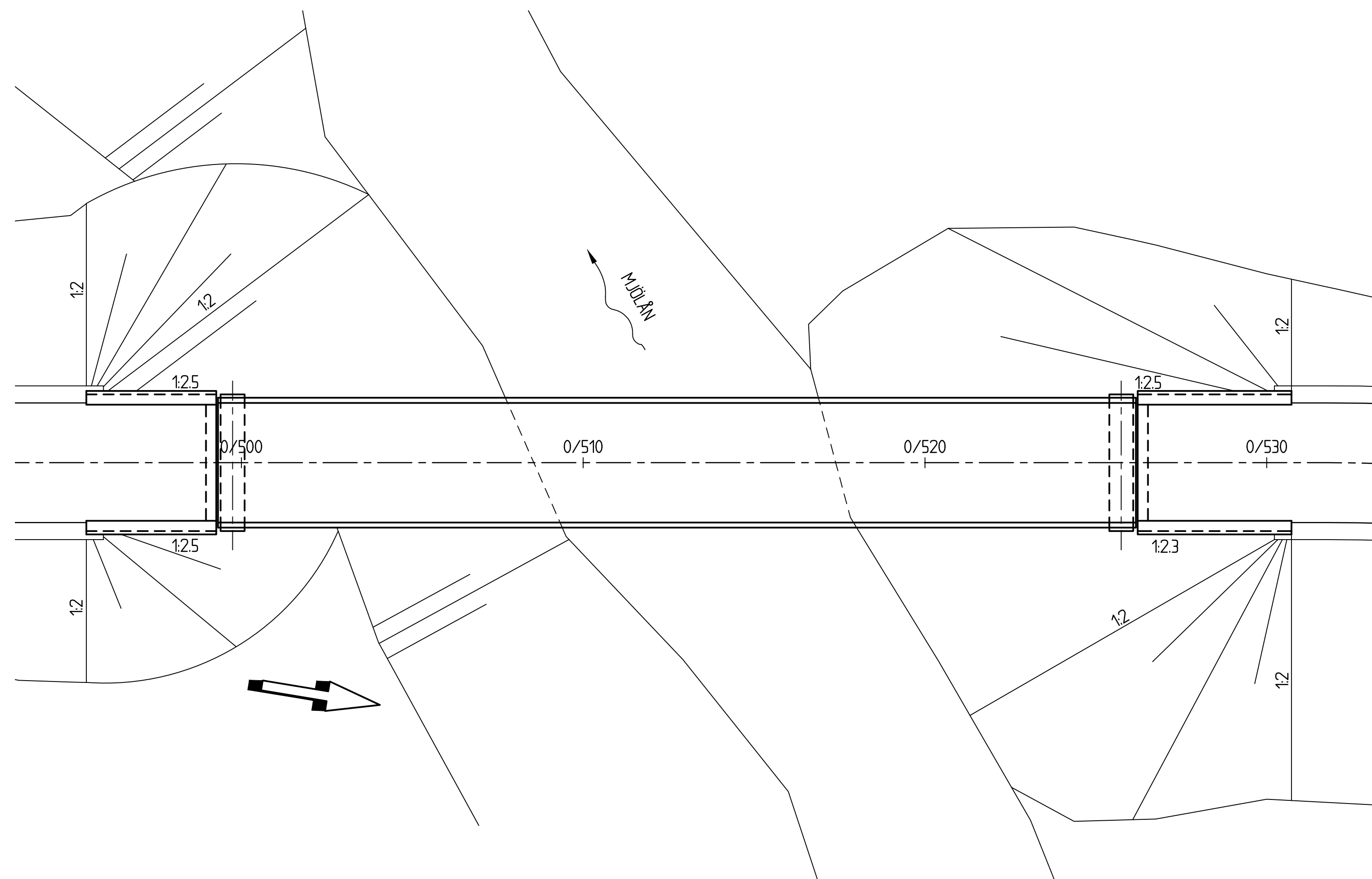
PLAN 1:100
