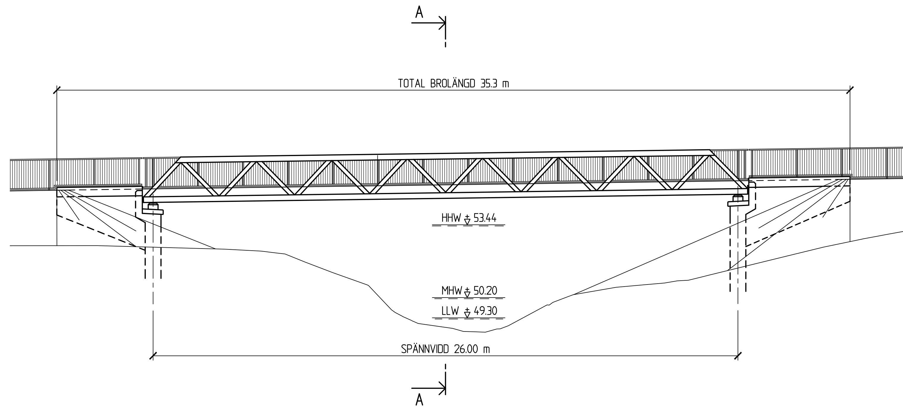
ELEVATION 1:100
