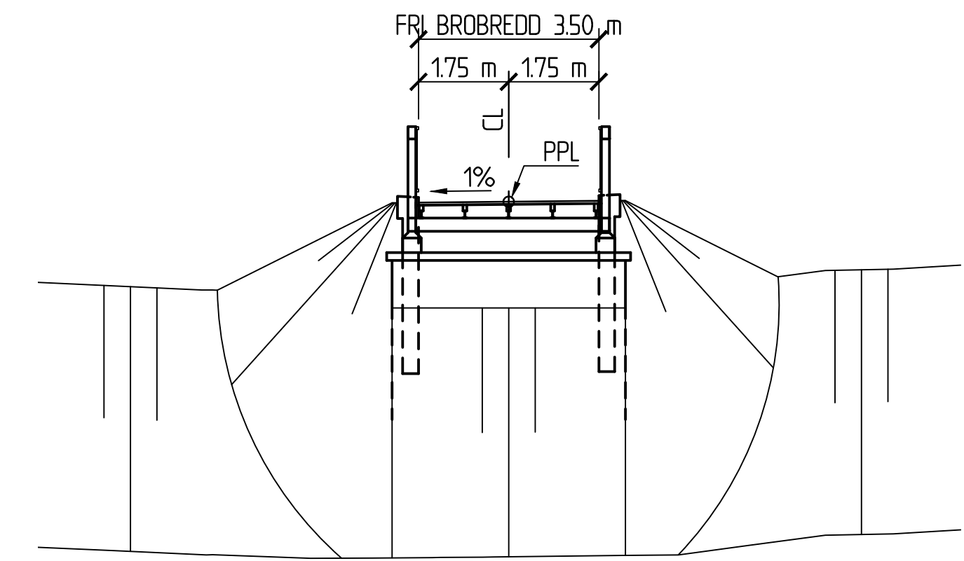
SEKTION A-A 1:100
