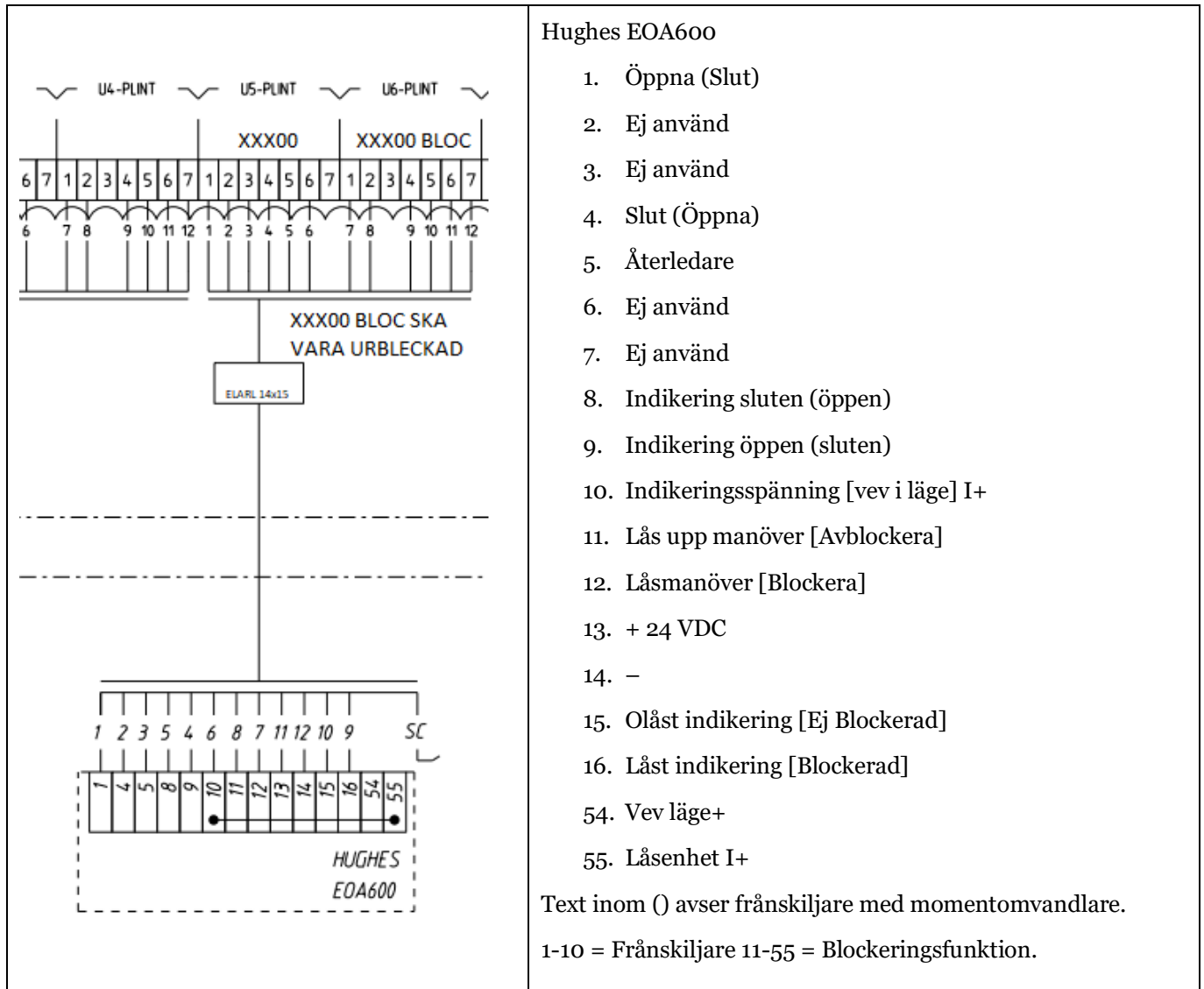
Figur 1 Kopplingschema Hughes EOA600 v3 (TRV artikel nummer: 9836720)
