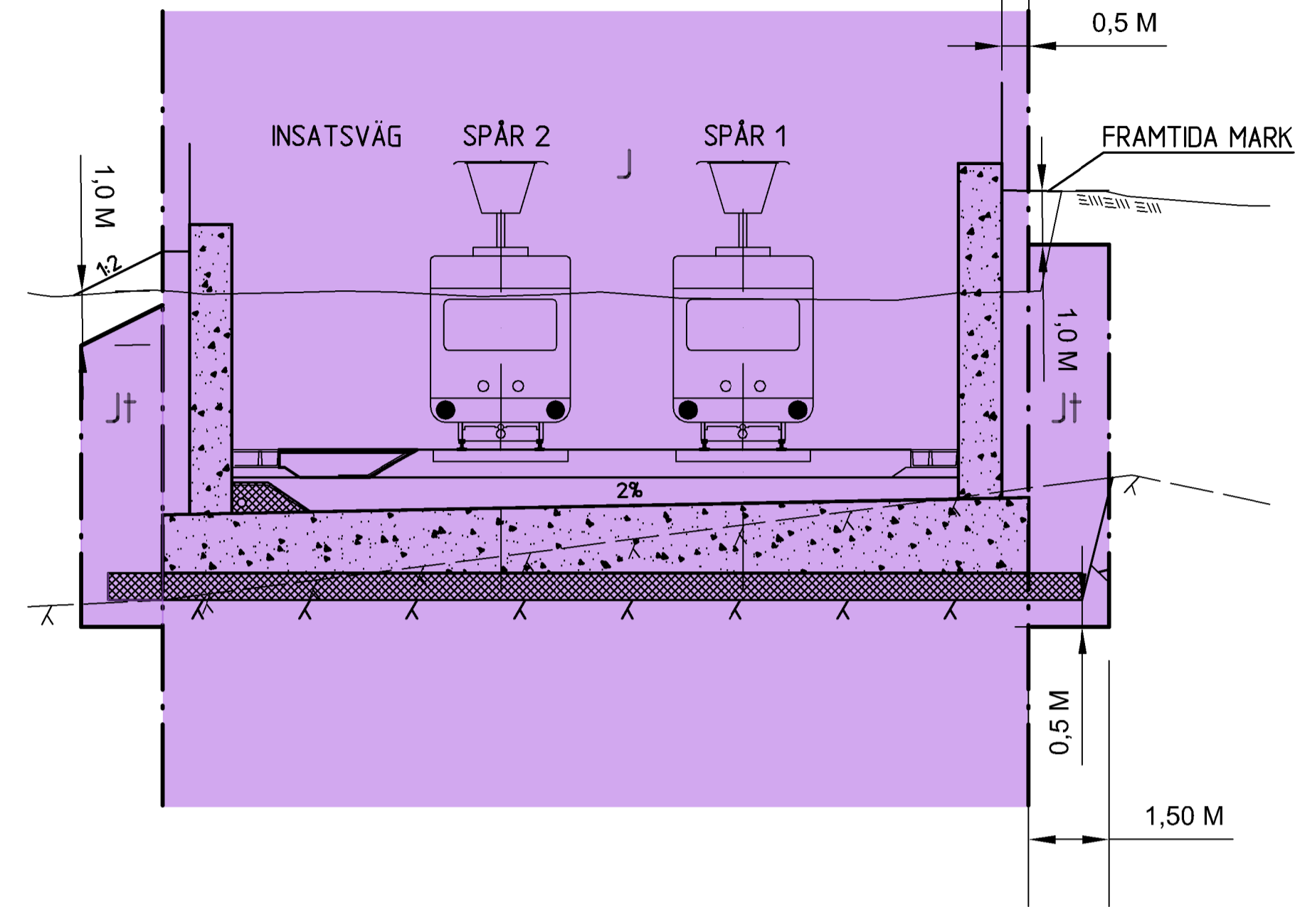
TYPSEKTION, NYTT DUBBELSPÅR I TRÅG
