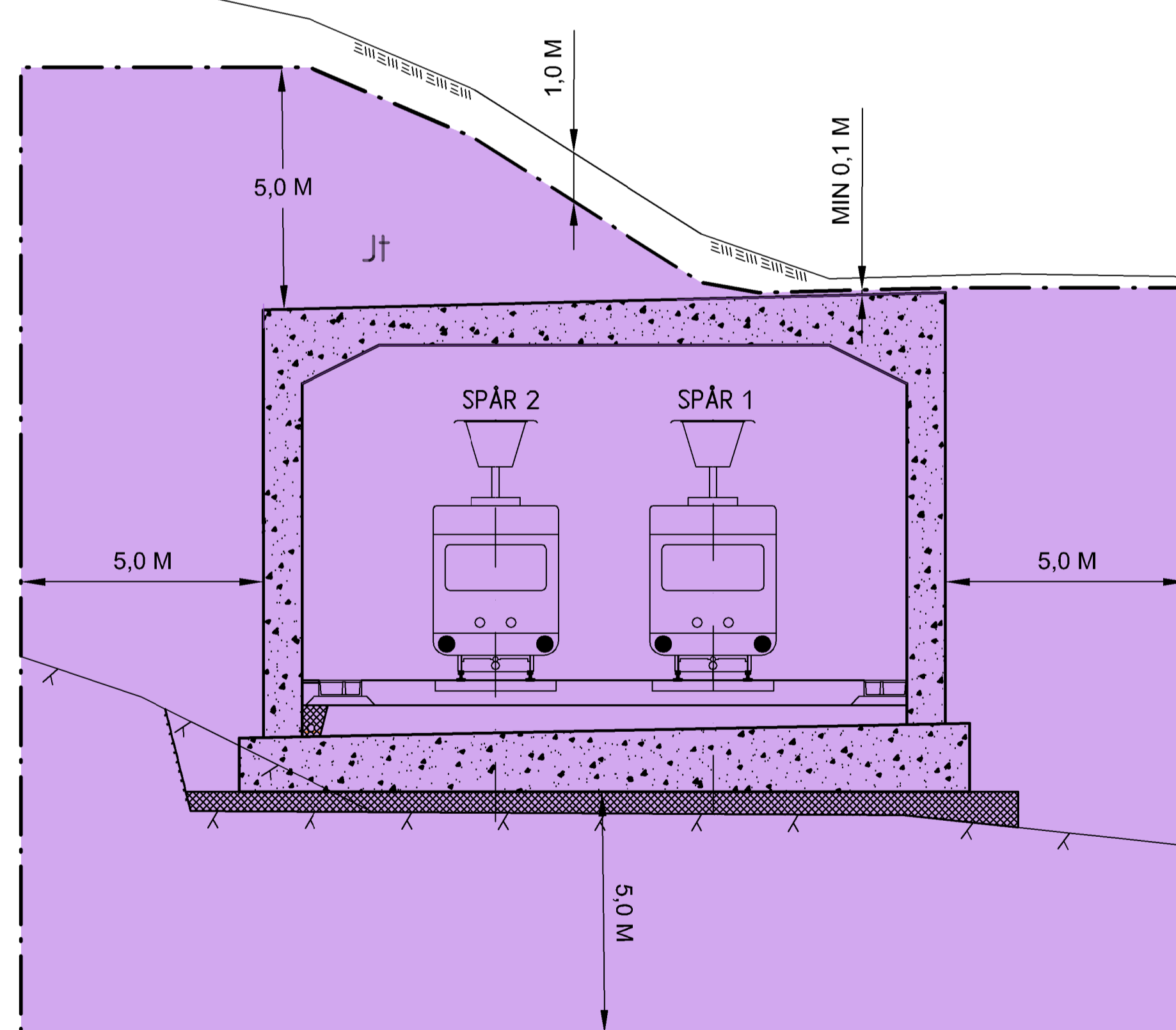
TYPSEKTION, NYTT DUBBELSPÅR I BETONGTUNNEL
