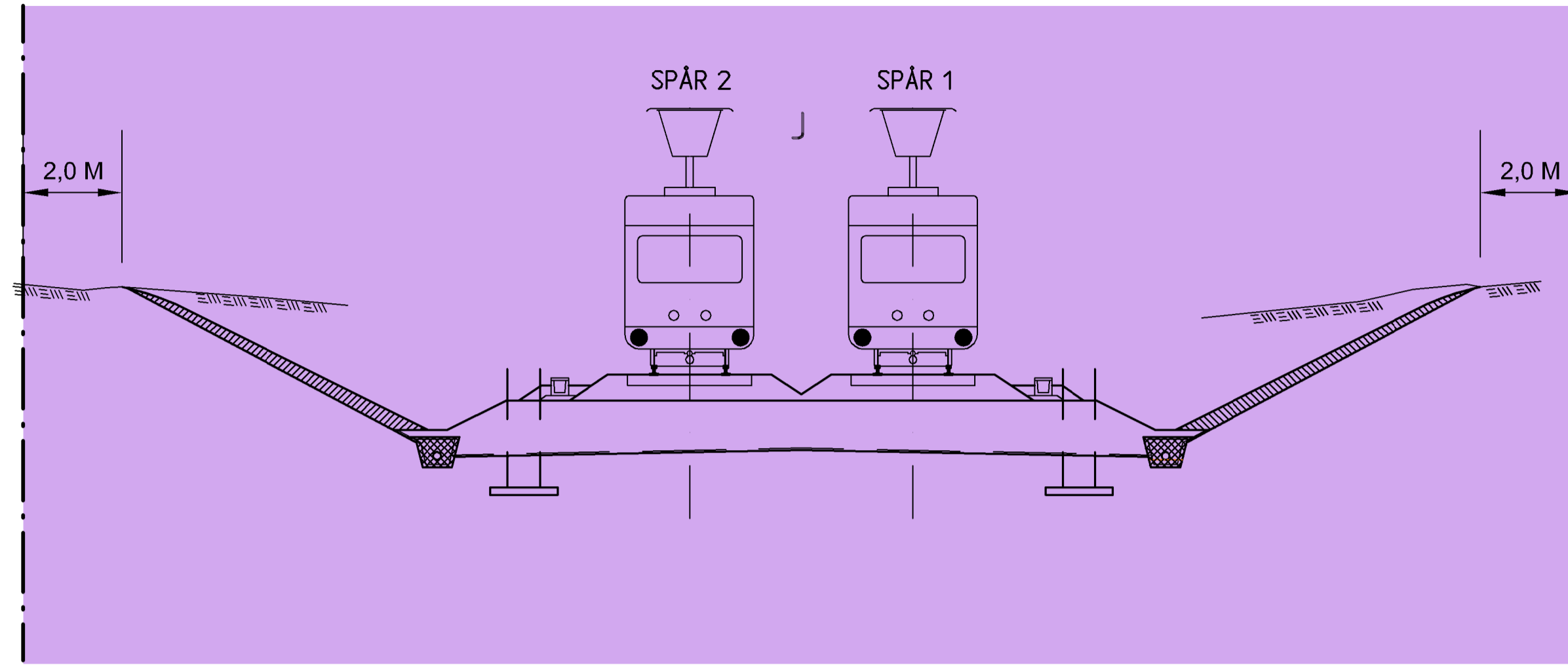
TYPSEKTION, NYTT SPÅR INTILL BEFINTLIGT, JORDSKÄRNING
