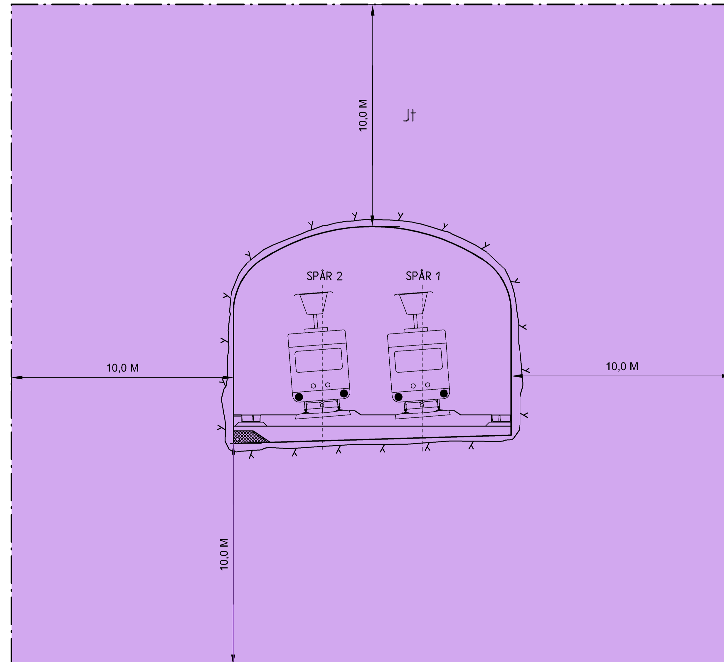
TYPSEKTION, NYTT DUBBELSPÅR I BERGTUNNEL
