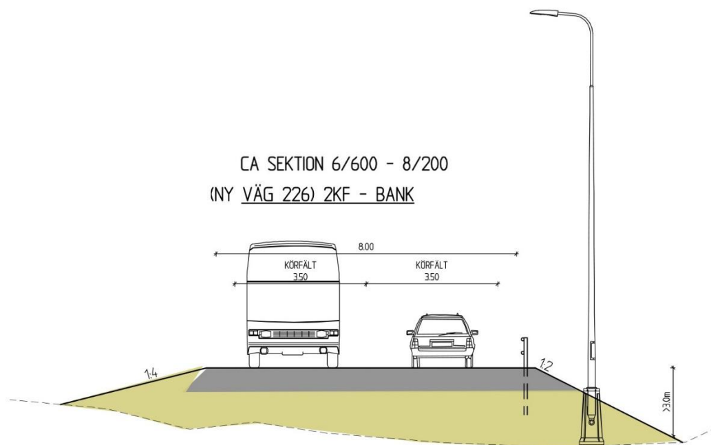
Figur 16. Sektion 2 körfält mellan Pålamalmsvägen – Hantverksbyn
