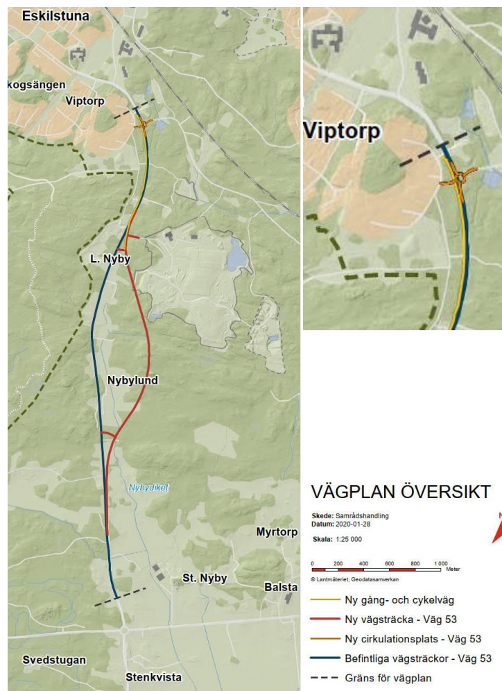
Figur 1. Ändringar i vägplan. Illustration: Tyréns AB.
