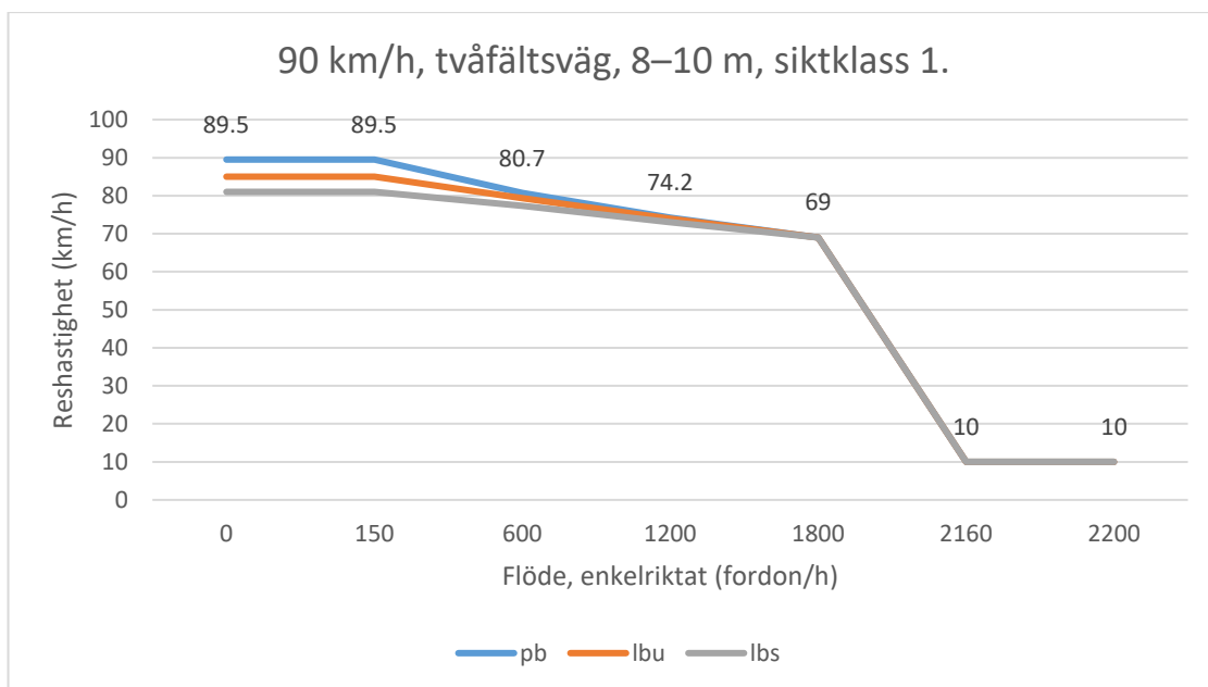
Figur 3. VQ-samband för 9 m väg siktklass 1. Hastighet för personbilstrafik redovisas i figuren för olika brytpunkter avseende totalt flöde (personbilstrafik+ lastbilstrafik med och utan släp)
