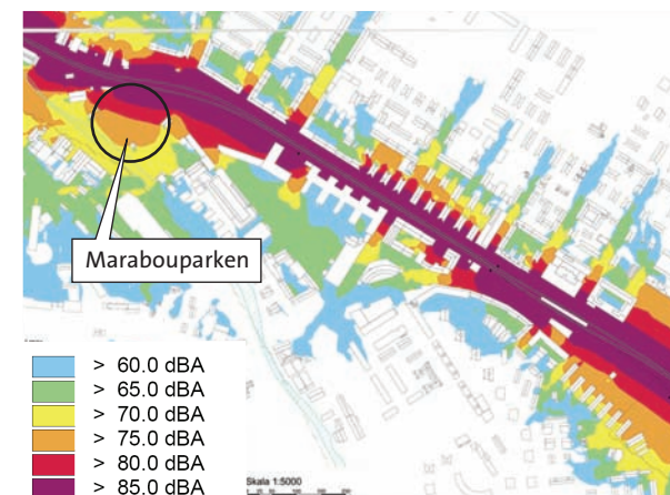
Nollalternativet i Sundbyberg, utomhus utan åtgärder. Maximal ljudnivå högre än 70 dBA inom och innanför gult område.
