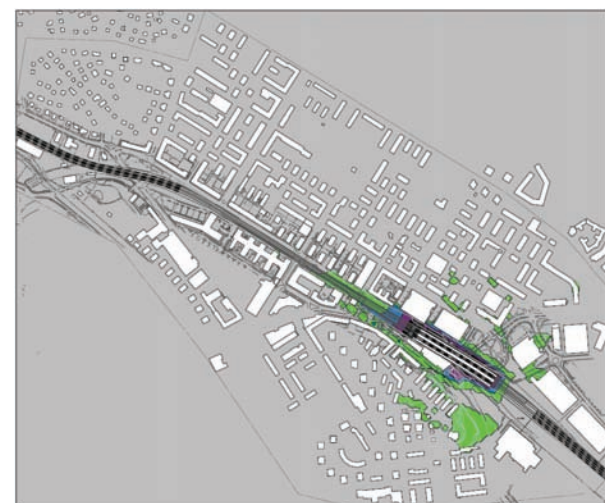
Skillnad mellan Tunnel med öppen station (utan skärm och överkragnig) och Tunnel med täckt station. Maximal ljudnivå (avser nivåer över 55 dBA) utomhus utan åtgärder.
