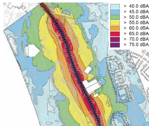
Utbyggnadsalternativ i Görvälns naturreservat, utomhus utan åtgärder. Ekvivalentnivå högre än 55 dBA inom och innanför gult område.
