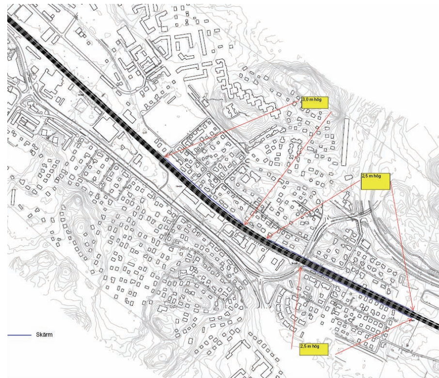
Befintliga bullerskärmar på sträckan genom Bromsten.
