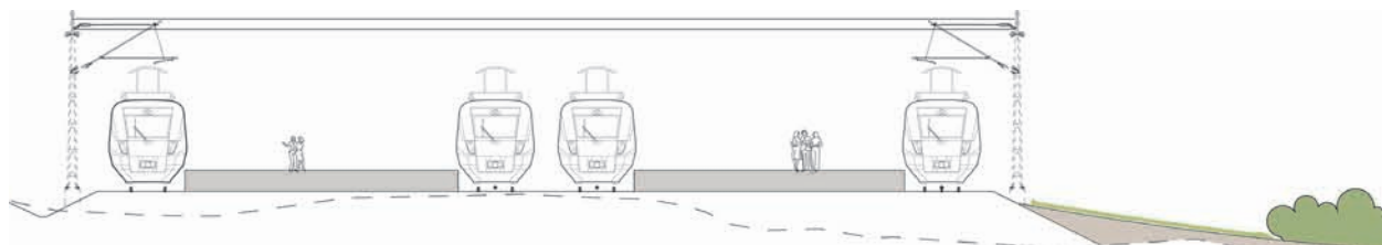
Förslag till utformning av en regionaltågsstation vid Barkarby med två mellanplattformar
