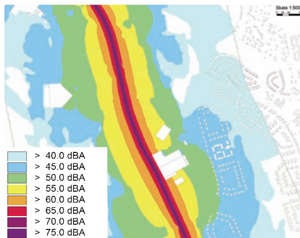
Nollalternativet i Görvälns naturreservat, utomhus utan åtgärder. Ekvivalentnivå högre än 55 dBA inom och innanför gult område.
