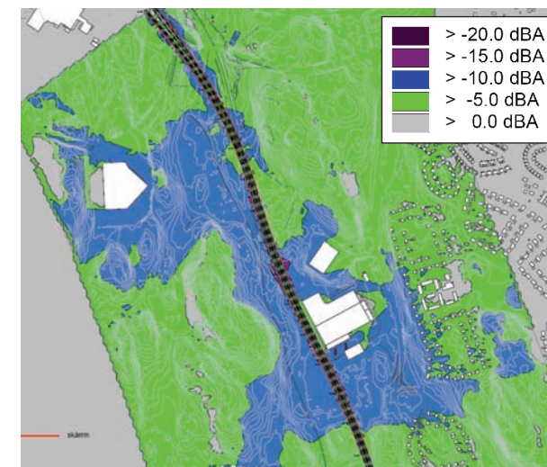
Utbyggnadsalternativ i Görvälns naturreservat, utomhus utan åtgärder. Skillnad mellan utbyggnadsalternativ i ekvivalent ljudnivå utan respektive med 2.5 meter höga skärmar genom Görvälns naturreservat, redovisat på båda sidor om spåren. Avser nivåer över 35 dBA.
