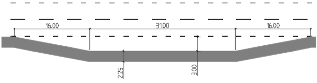
Figur 20. Fickhållplats i plan.
