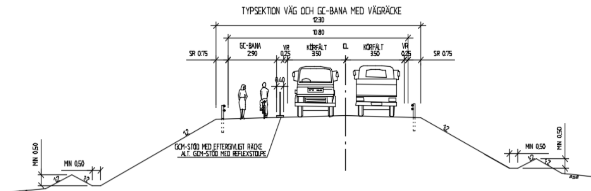
Figur 16. Typsektion på ny väg och GC-bana med vägräcke. SR= stödremсор och VR=vägren.
