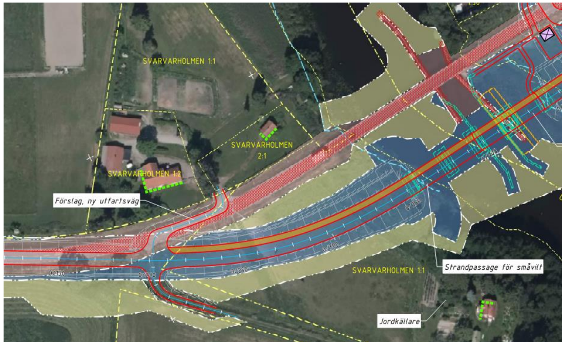
Figur 18. Enskilda anslutningar på södra sidan om bron.
