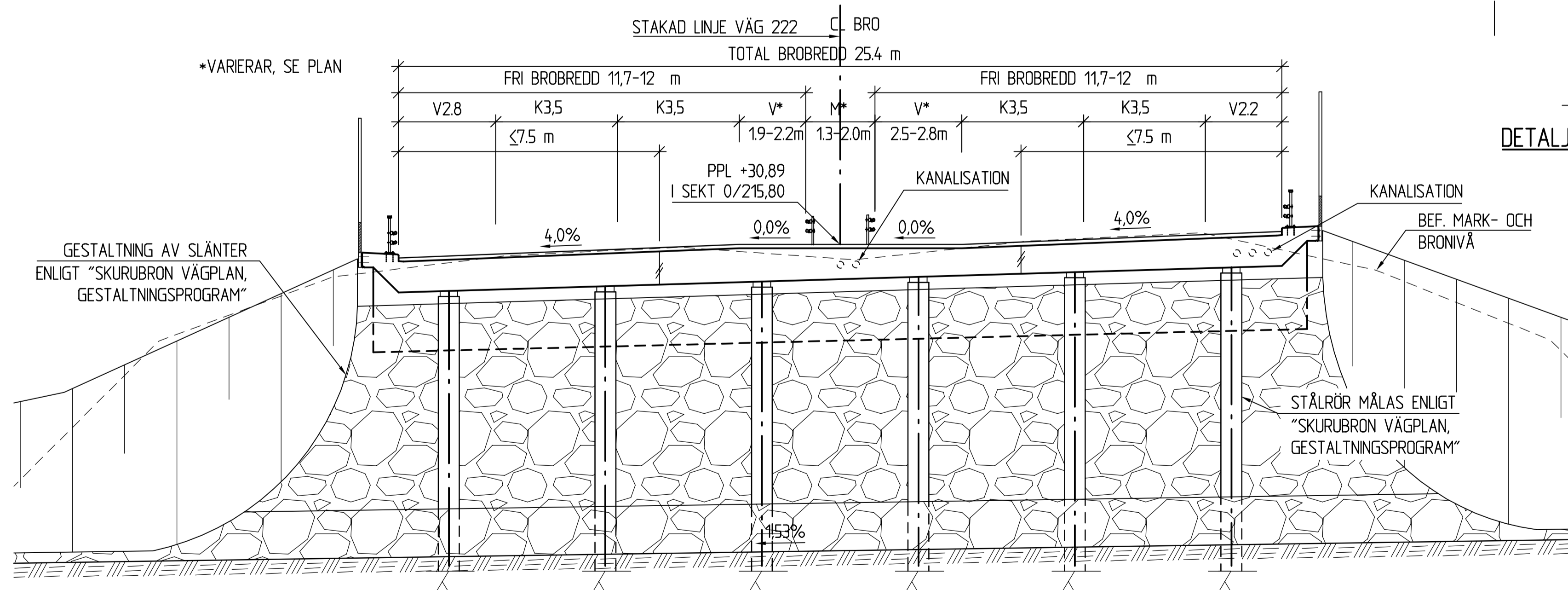
SEKTION B-B SKALA 1:100
