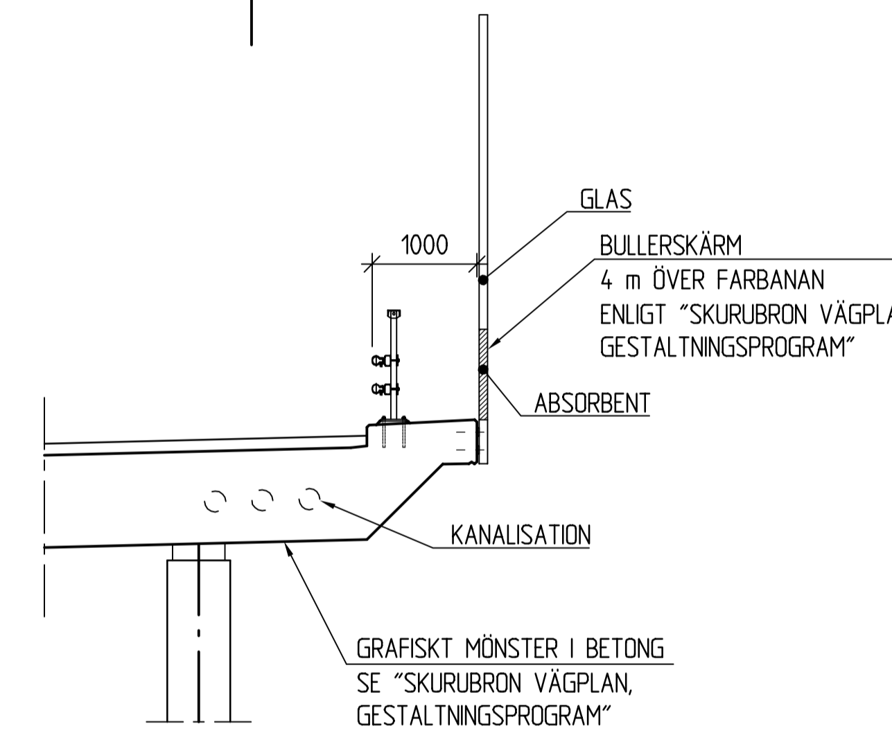
DETALJ 1 SKALA 1:50
