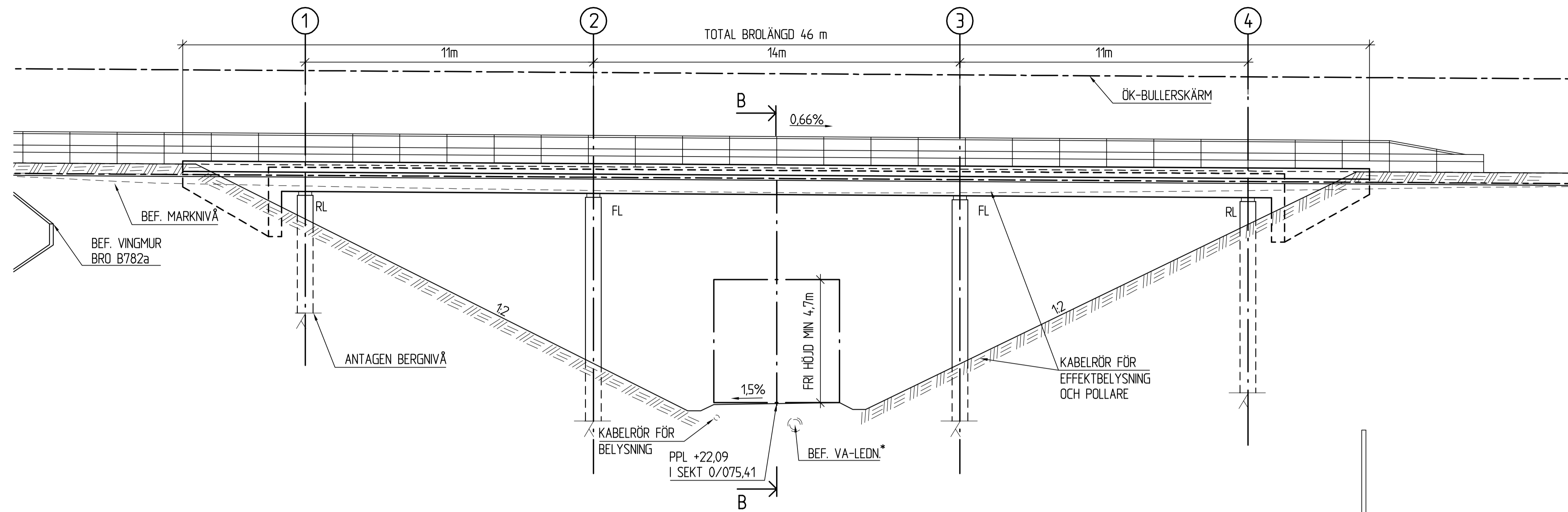
ELEVATION SKALA 1:100
