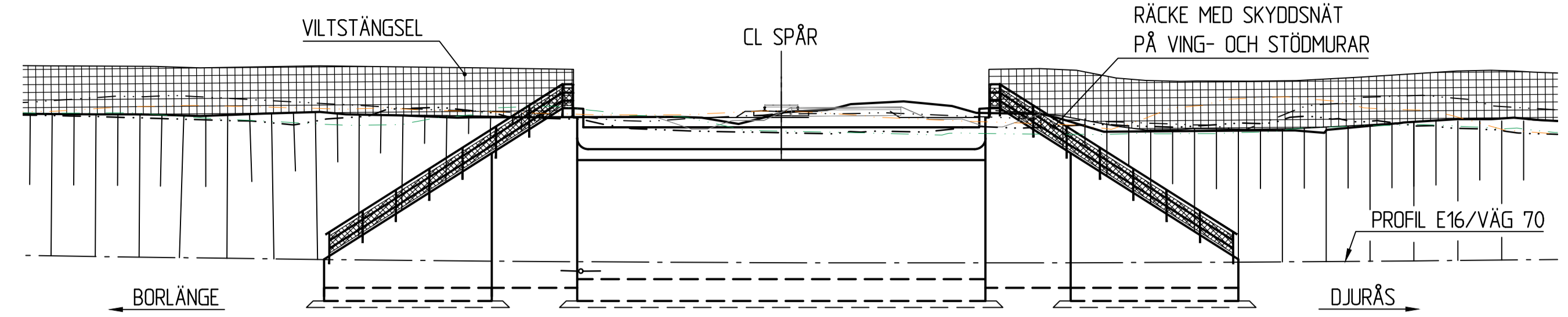
SEKTION B-B 1:200
