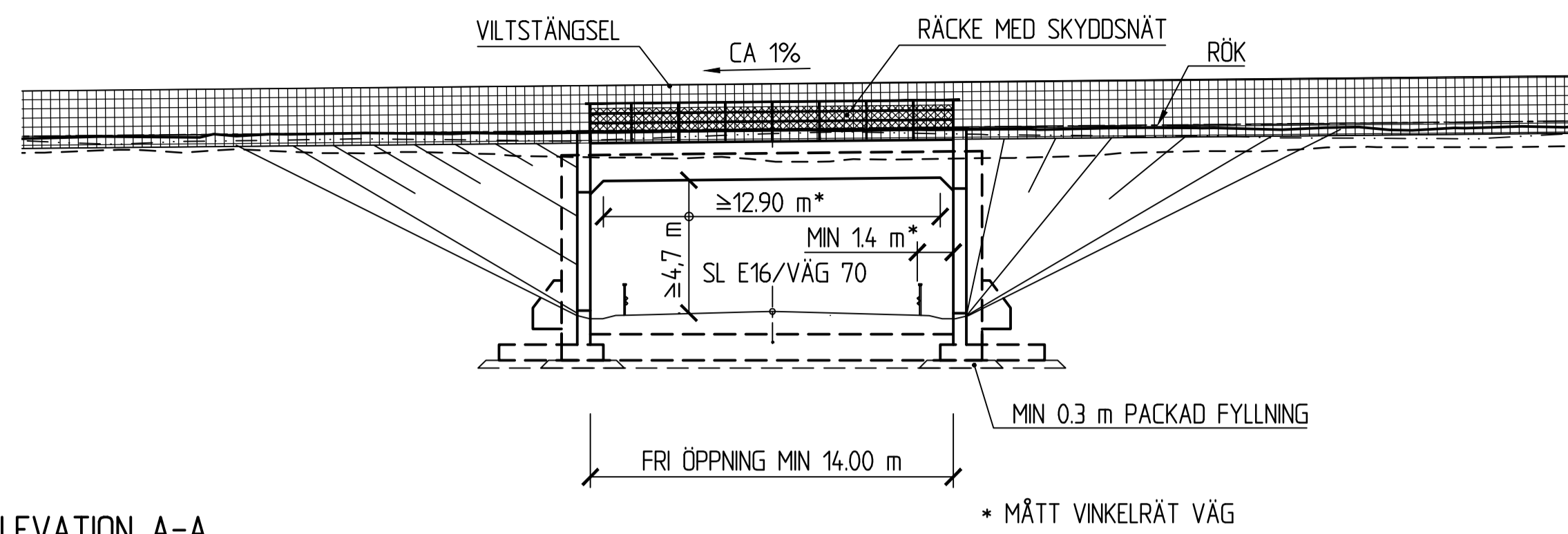
ELEVATION A-A 1:200
