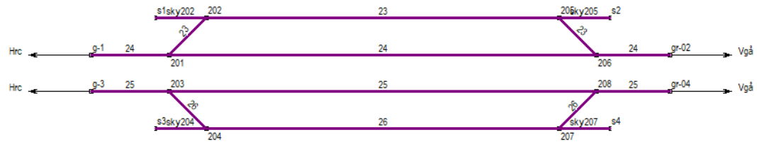
Figure 1 Track layout Herrljunga västra
