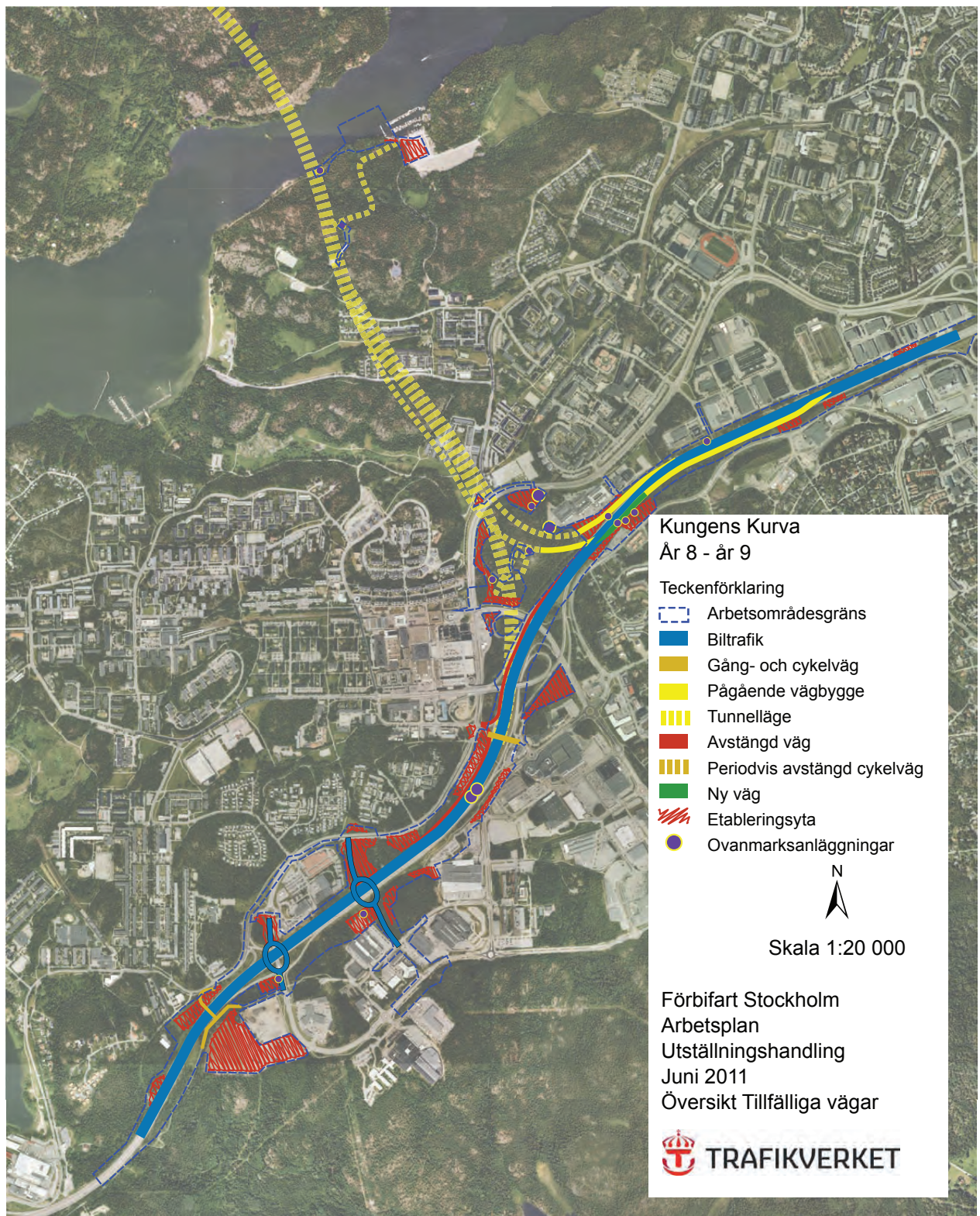
Figur 1.25 Ett studerat alternativ till trafikföring under byggnadstiden. Kungens kurva år 8-9 I den sista etappen byggs bergtunnelanslutningen med E20 österifrån. Omläggningen av trafiken sker på den norra delen av nuvarande E4/E20
