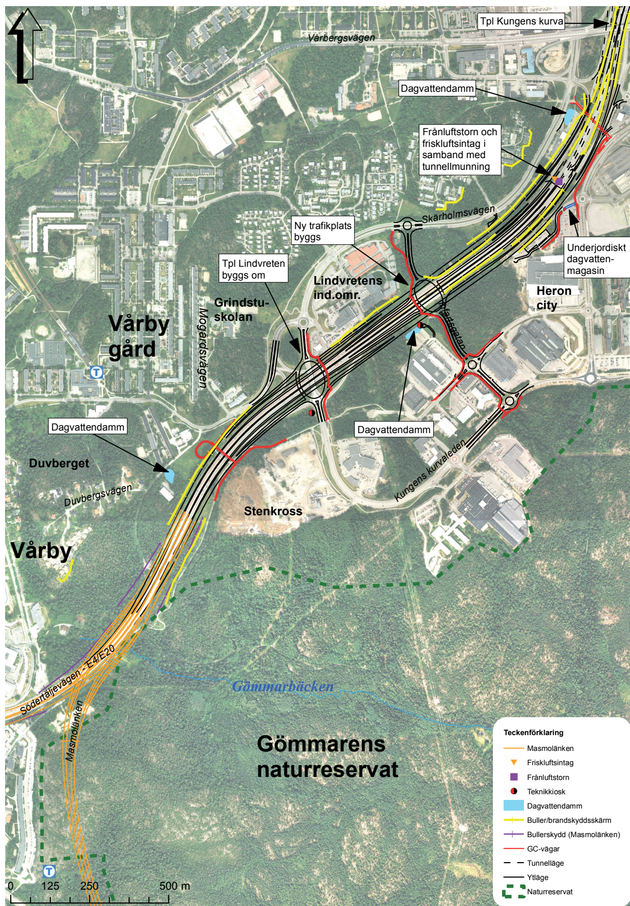
Figur 1.13 Skadeförebyggande åtgärder. Skyddsskärmar redovisas på illustrationsritningar i denna pärm
