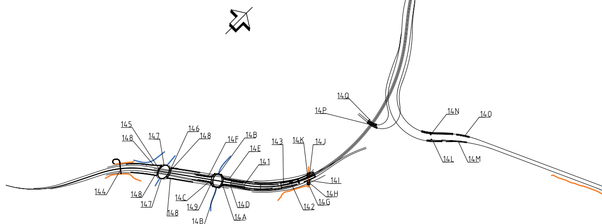
Figur 1.12 Beteckningar på byggnadsverk, se även tabell 1.5. Gång- och cykelvägar anges i orange och kommunala vägar i blått.r
