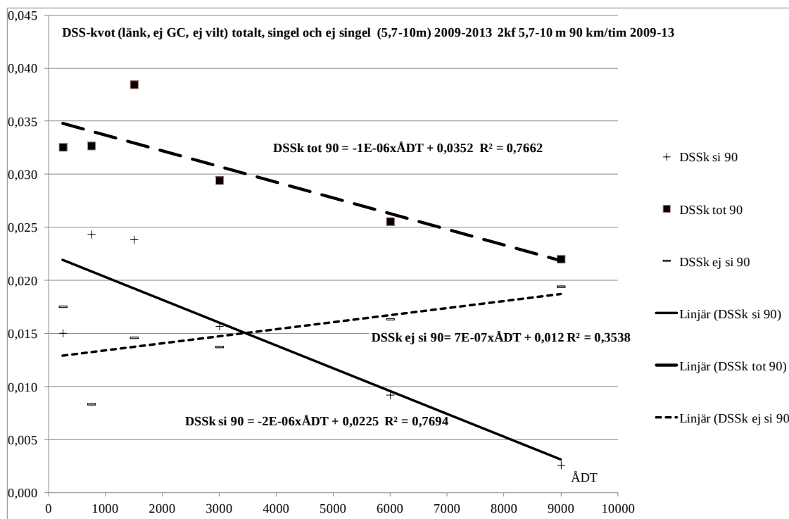
Figur 2: Empiri (2009-2013) antal dödade och svårt skadade totalt, i singel och ej singel i mf/mf- och mf/singelolyckor vid olika ÅDT på tvåfältsväg (5,7-10m) landsbygd 90 km/tim.
