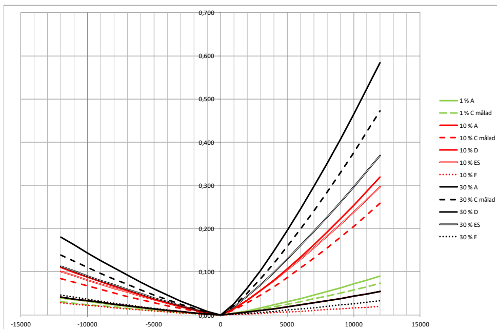
Figur 27 DSS år 2010 för 3-vägs- och likafördelade 4-vägs korsningar med olika andel inkommande sekundärvägstrafik vid 70 km/h i landsbygdsmiljö.
