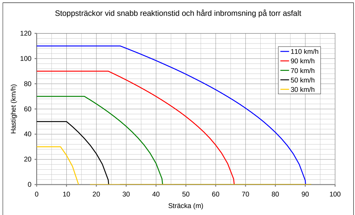
Figur 23 Stoppträckor för personbil vid olika hastigheter med 1 sek reaktionstid.
