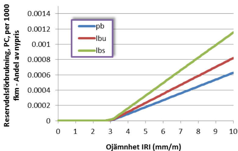
Figur 7 Reservdelsförbrukning, PC, som funktion av vägens jämnheter
