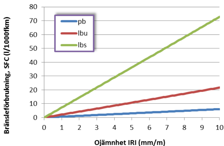
Figur 6 Relativ bränsleförbrukning som funktion av vägens jämnhet för personbil(pb), lastbil utan släp (lbu) och lastbil med släp (lbs) då ingen hänsyn tas till hastighetsförändring.
