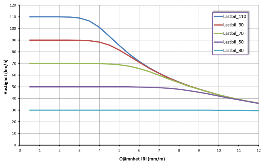
Figur 5 Samband hastighet och ojämnhhet för lastbilar
