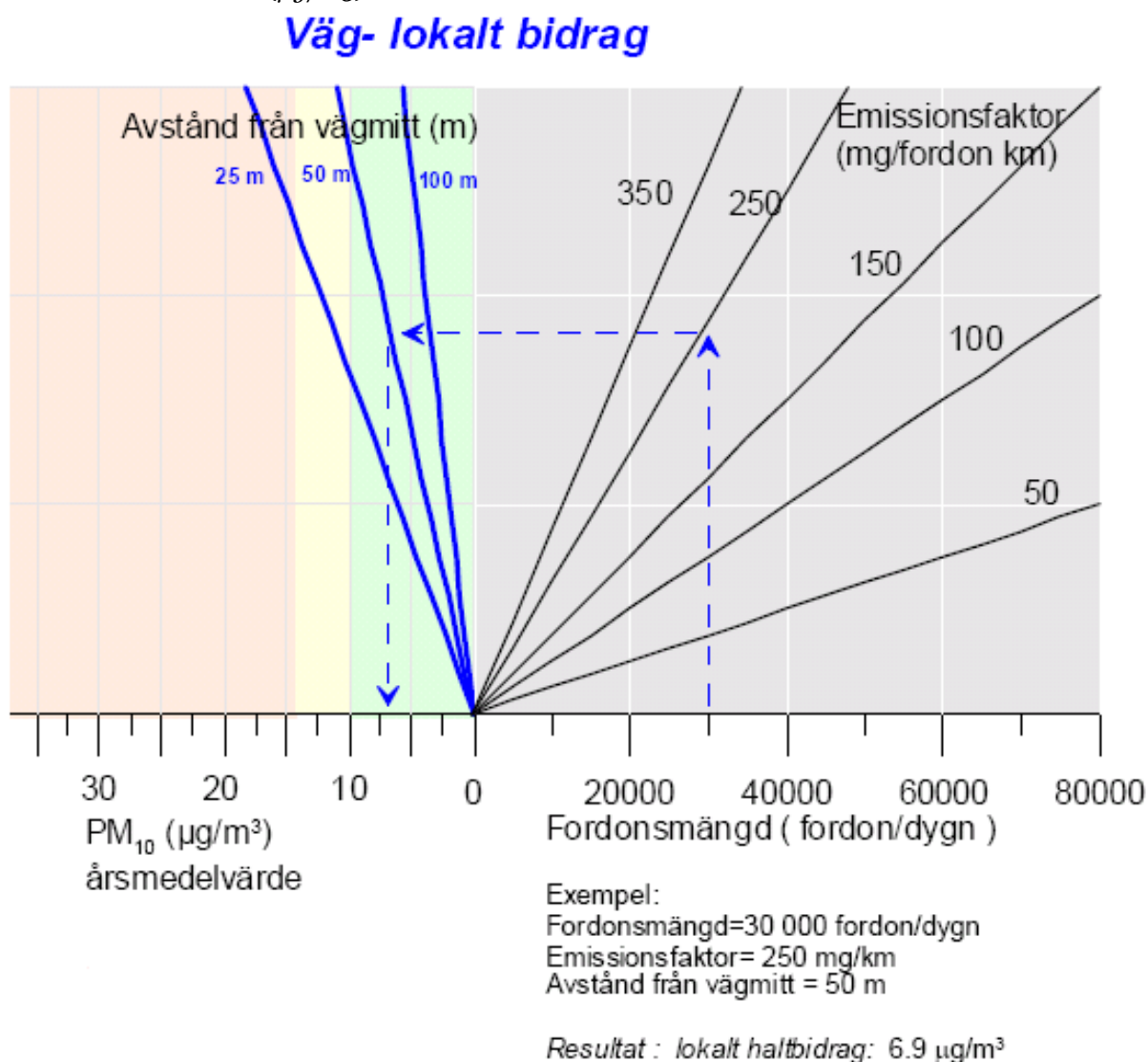
Figur 11 Nomogram för beräkning av lokala bidrag från gaturum till årsmedelhalter av PM 10 ( \mu\text{g}/\text{m}^3 )
