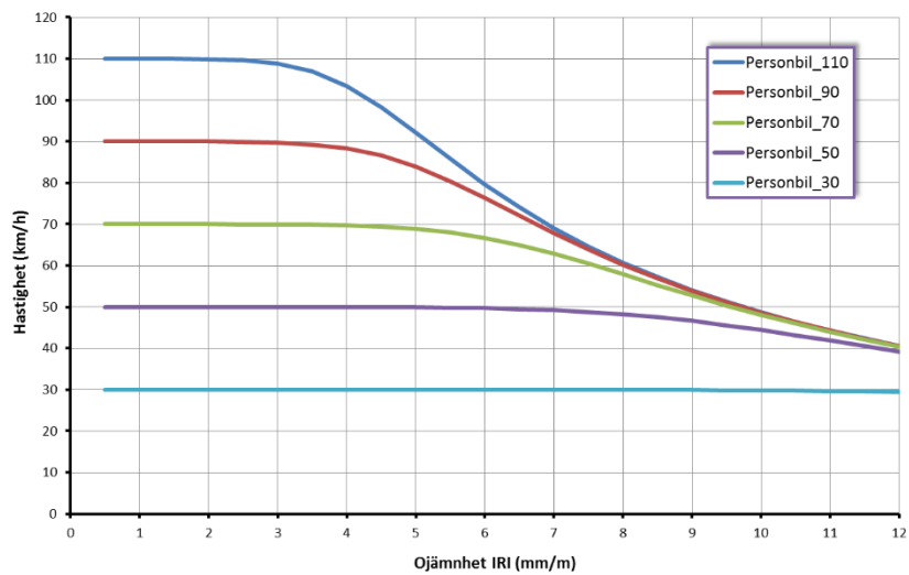
Figur 4 Samband hastighet och ojämnhhet för personbilar
