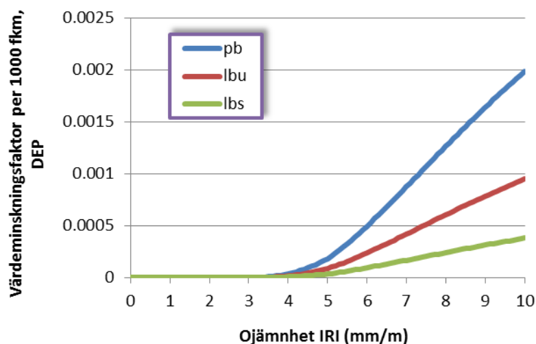
Figur 9 Värdeminskning som funktion av vägens jämnhet
