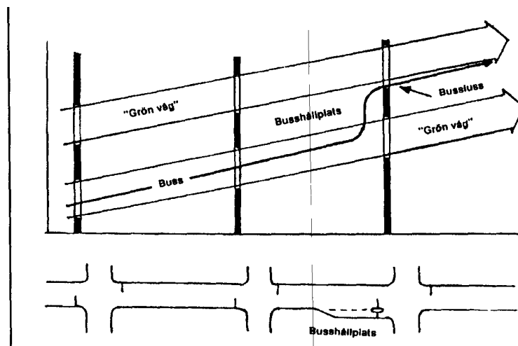
Figur 10.9. Exempel på lämplig placering av hållplats vid passiv prioritering i samordnade trafiksignalssystem.
