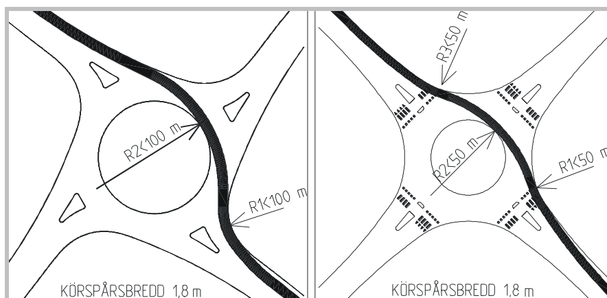
Figur 4-52 Körspårsradie i en cirkulationsplats.
