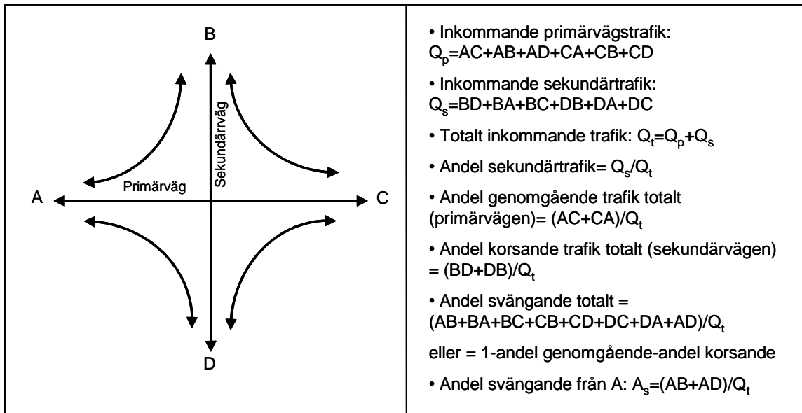
Figur 4-9. Trafikbegrepp i korsningar.
