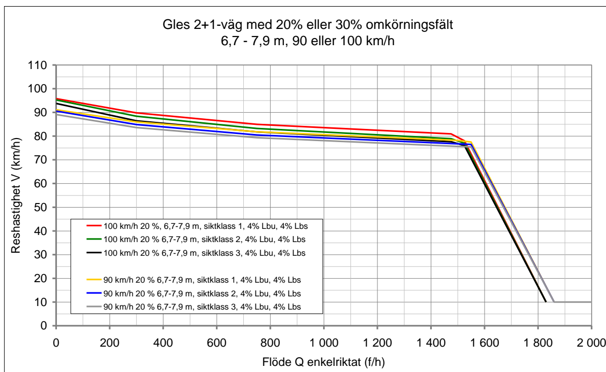
Figur 4-49. Reshastighetflödessamband (VQ) för 6,7 – 7,9 m bred gles 2+1-väg med hastighetsbegränsning 90 eller 100 km/h. Vägarna har växlande 2,1 km (20%) eller 3,6 km (30%) enfältsavschnitt och 0,9 km omkörningsfält. 4% LBU och 4% LBS är genomsnittliga lastbilsandelar för Riksvägar och primära länsvägar.
