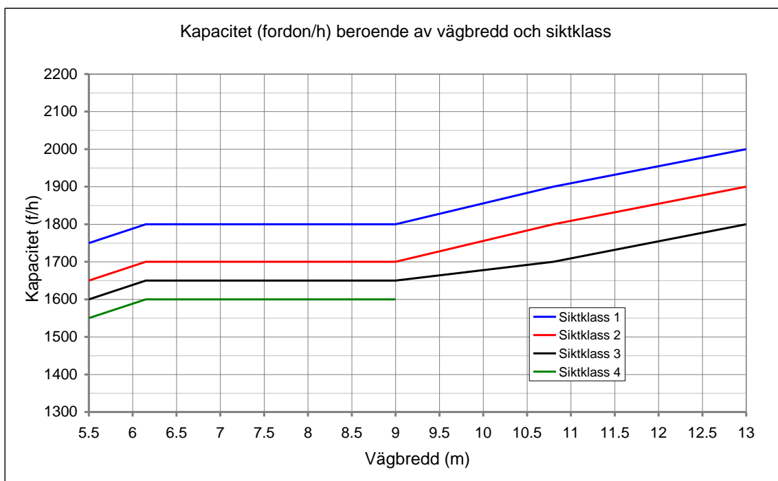
Figur 4-37. Kapacitet vid siktclass 1 och 4 för olika vägbredder.
