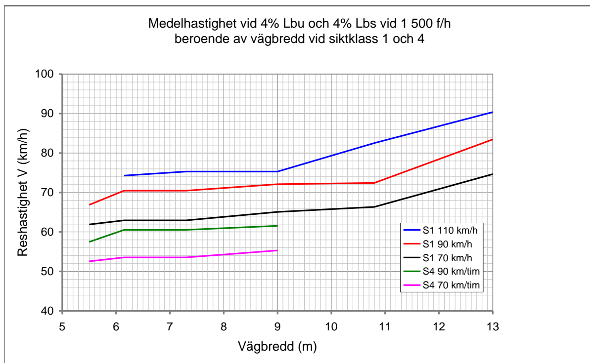
Figur 4-38. Medelhastighet vid siktclass 1 och 4 för olika vägbredder och hastighetsbegränsningar då belastningen är 1 500 f/h.
