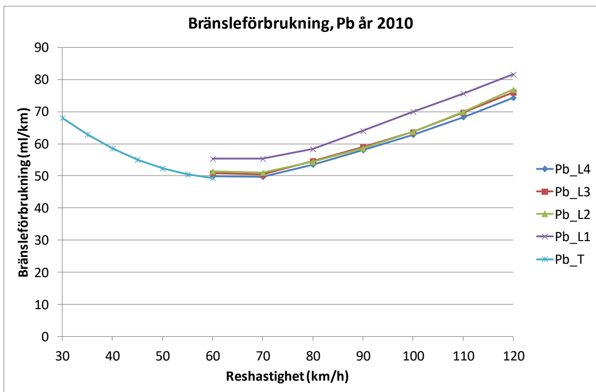
Figur 4-56. Bränsleförbrukning för personbil år 2010 för olika körförlopp.
