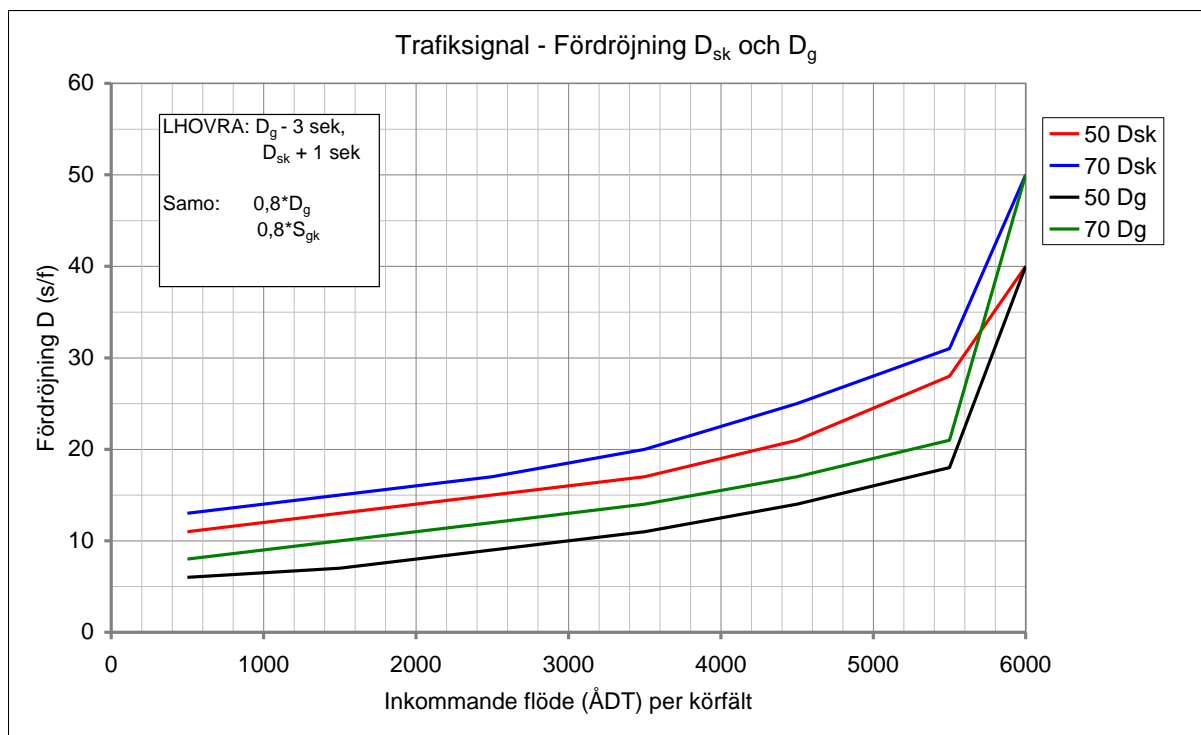
Figur 4-29. Fördröjning i korsning med trafiksinal.
