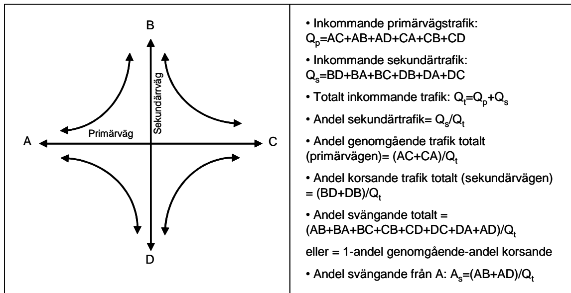
Figur 4-26. Trafik i korsningstyp A-C
