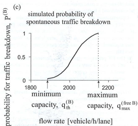
Figur 4-54 Sannolikhetsfördelning för risk för sammanbrott mellan min kapacitet och max kapacitet (Kerner, 2013) 57
