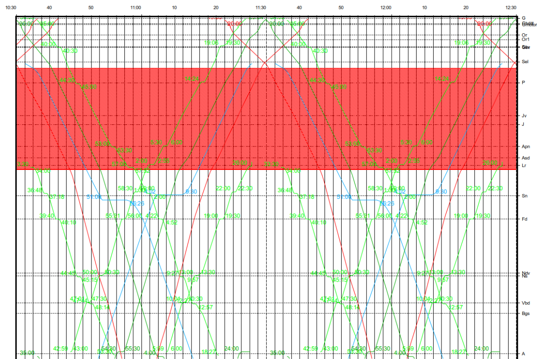
Figur 10. Principiell graf för sträckan Göteborg C – Alingsås under etapp 2, lågtrafik
