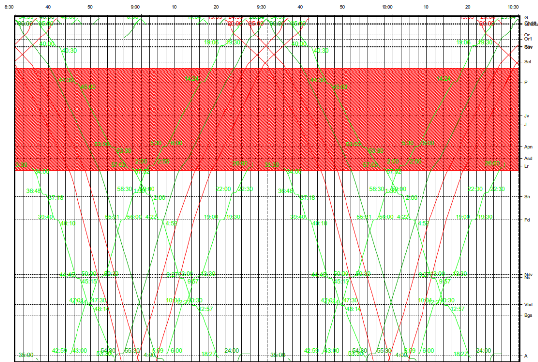
Figur 11. Principiell graf för sträckan Göteborgs central–Älvsjö under etapp 2, högtrafik
