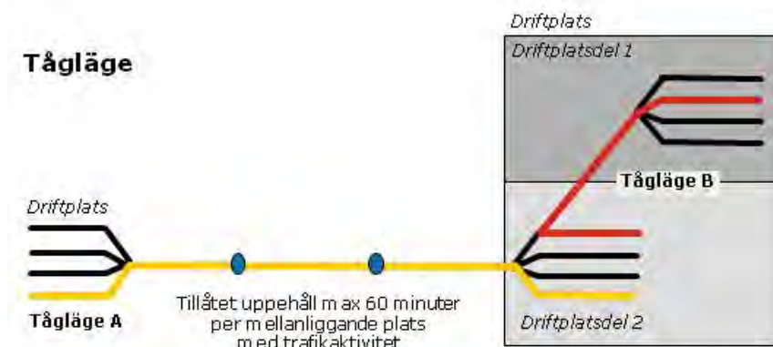
Figur 5.1 Tågläge alternativ A – mellan driftplatser. Tågläge alternativ B – mellan driftplatsdelar.
