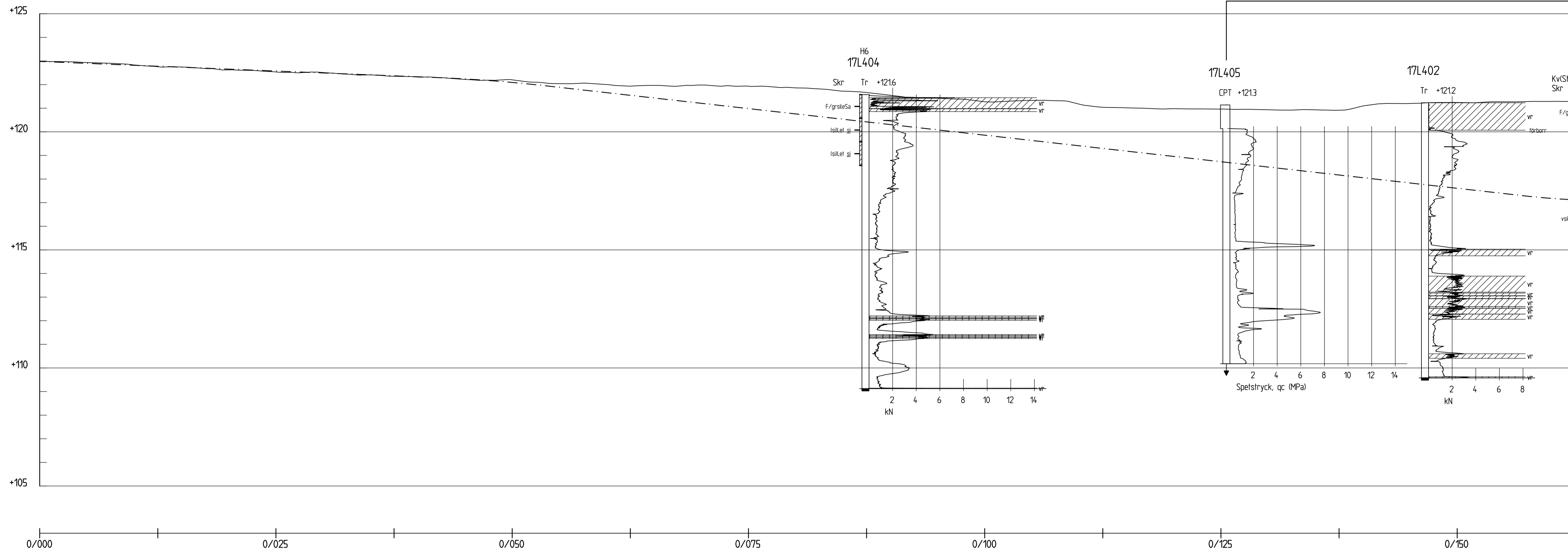
PROFIL H 1:100 L 1:250
