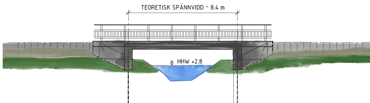
Figur 4.2 Föreslag konstruktionsskiss av gång- och cykelvägsbro över Flädiebäcken.
