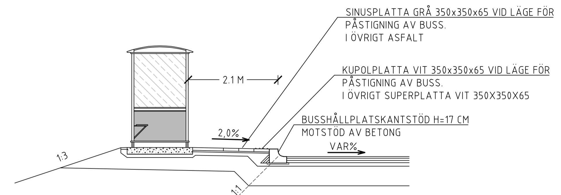
SEKTION A-A SKALA: 150
