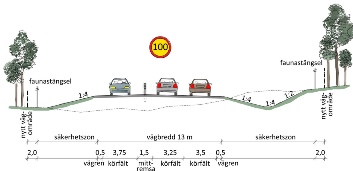
Figur 17. Typsektion Väg 27 2+1.
