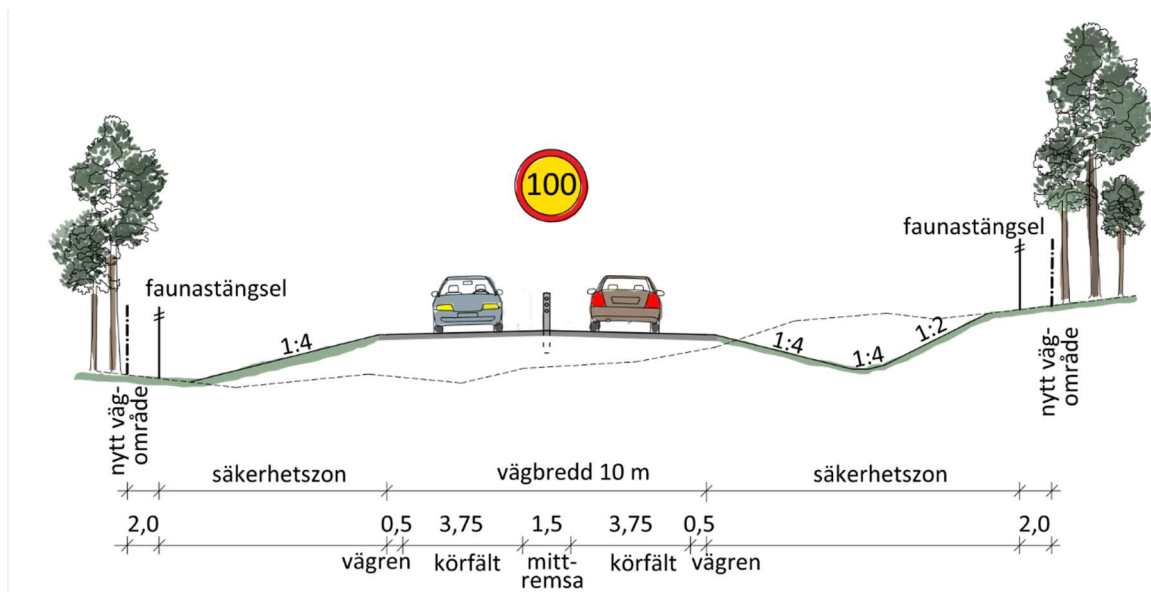
Figur 18. Typsektion Väg 27 1+1.
