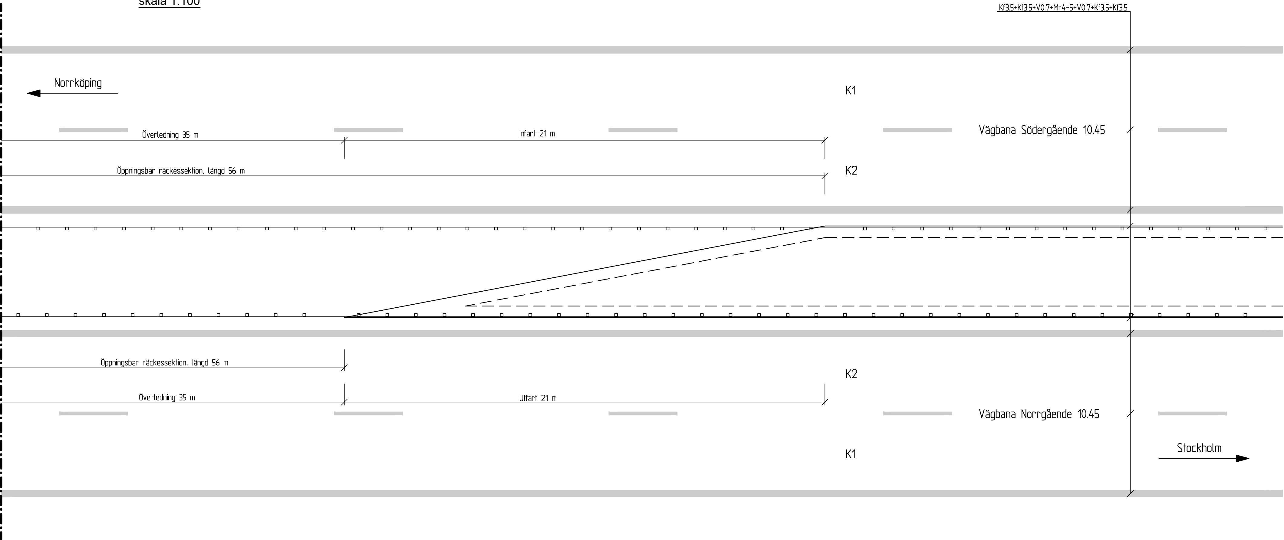
E4 Överledningsplats i mittremsa skala 1:100
