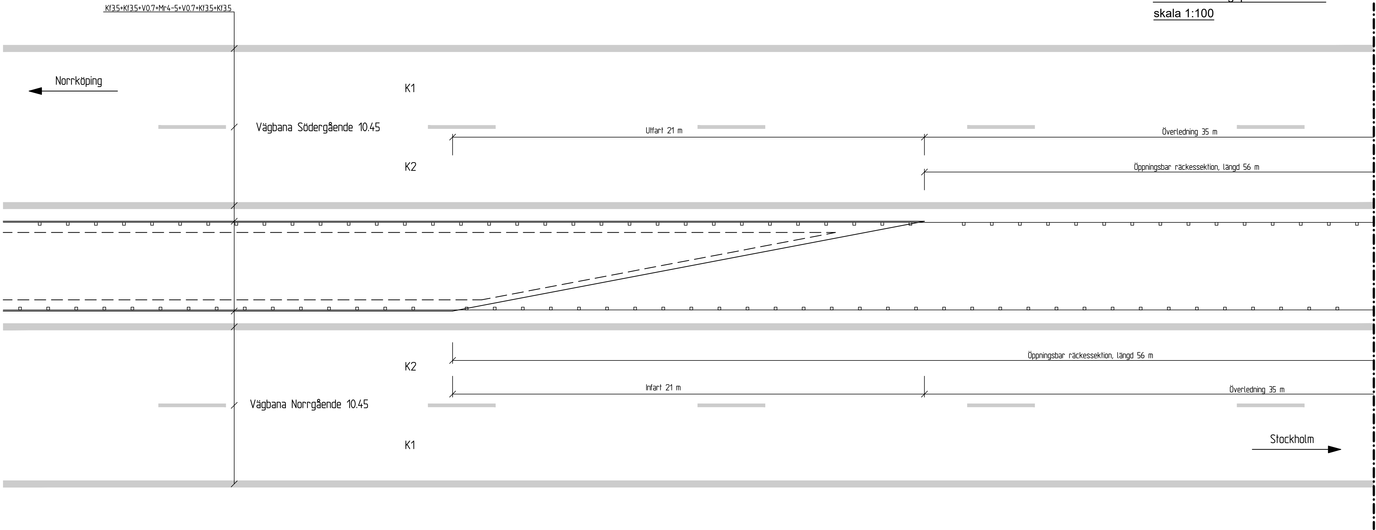
E4 Överledningsplats i mittremsa skala 1:100
