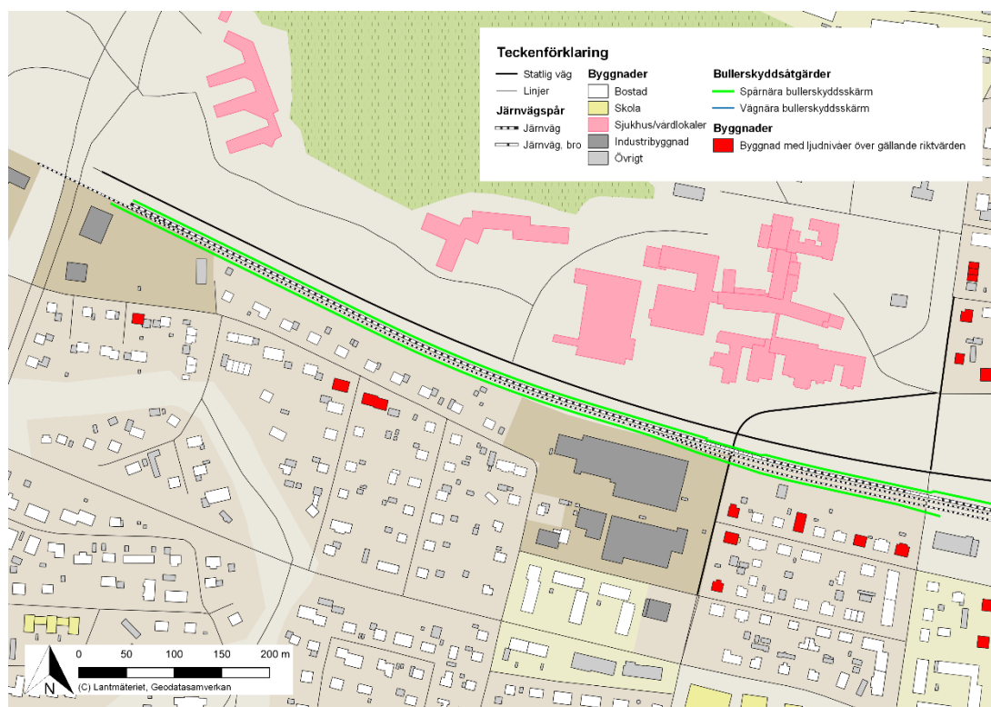
Figur 6.13: Byggnader med ljudnivåer över gällande riktvärden med spår- och vagnåra bullerskyddsåtgärder.
