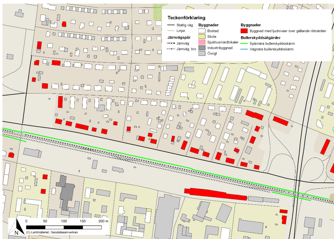
Figur 6.12: Byggnader med ljudnivåer över gällande riktvärden med spår- och vagnnära bullerskyddsåtgärder.
