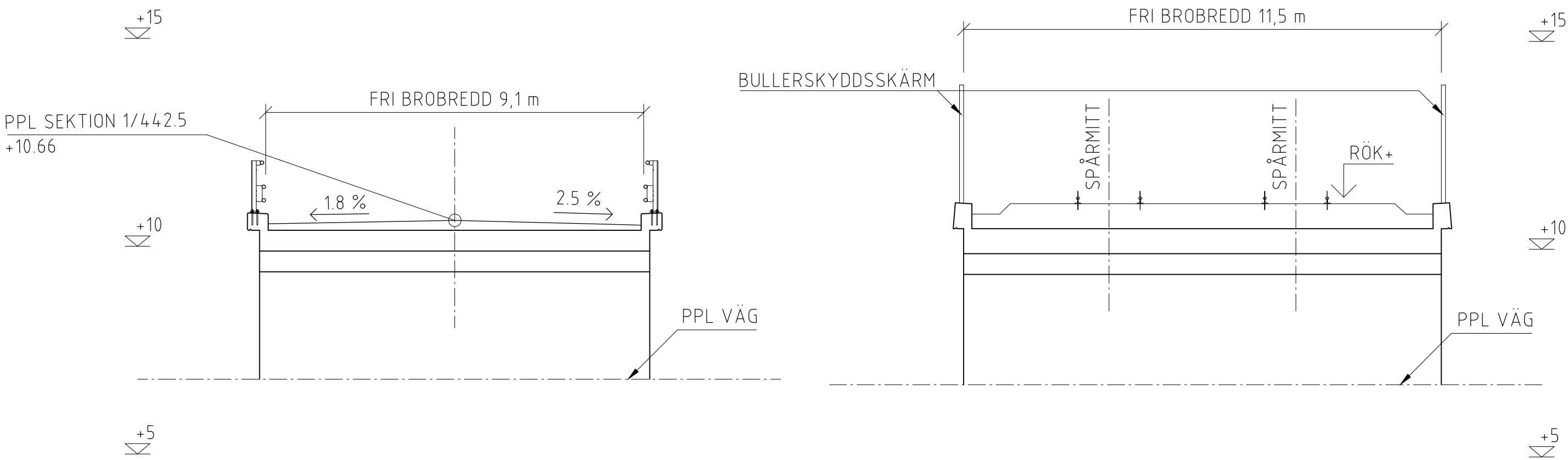
SEKTION D-D SKALA 1:100 JVG-BRO
