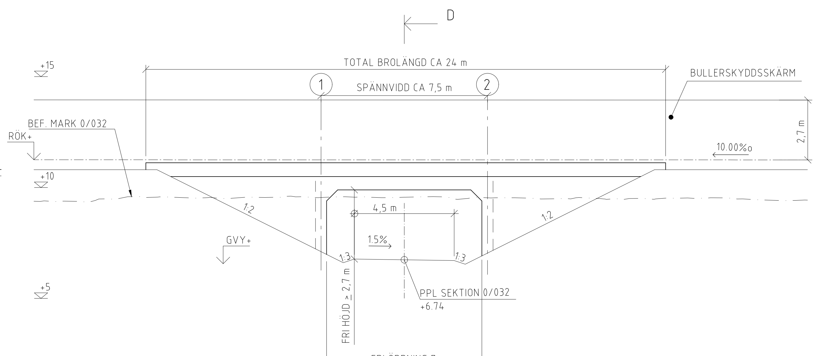
ELEVATION C-C SKALA 1:100 JVG-BRO
