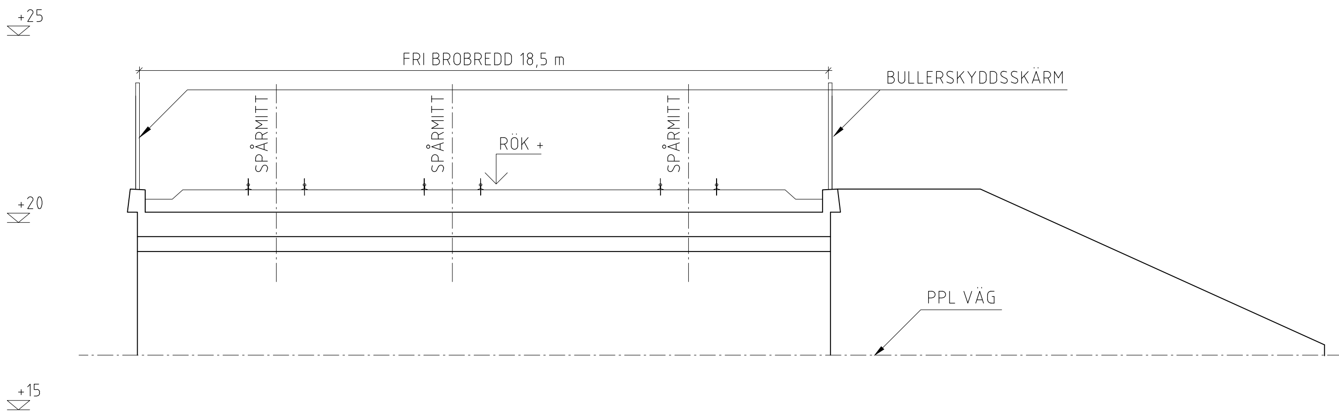
SEKTION B-B SKALA 1:100
