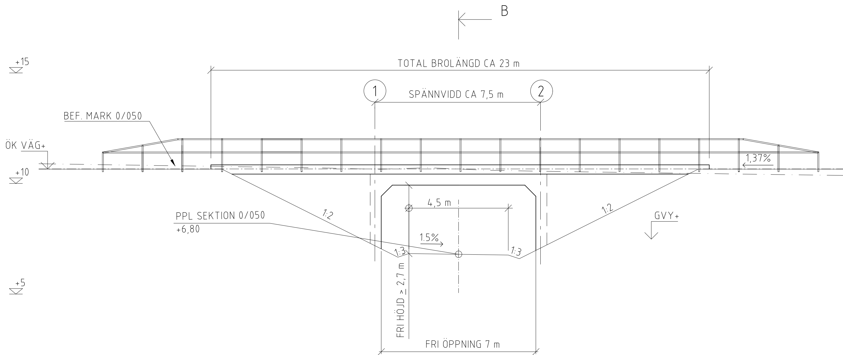
ELEVATION A-A SKALA 1:100 VÄGBRO
