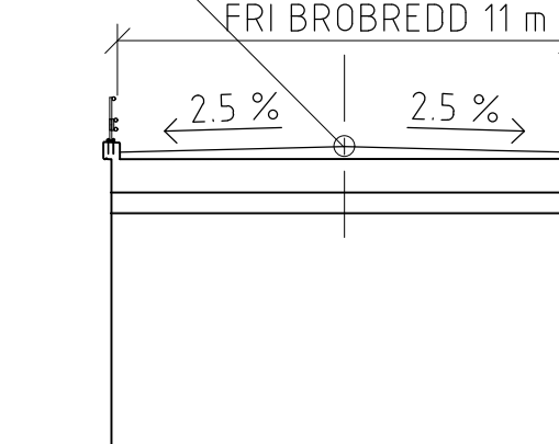
SEKTION D-D SKALA 1:200 VÄGBRO
