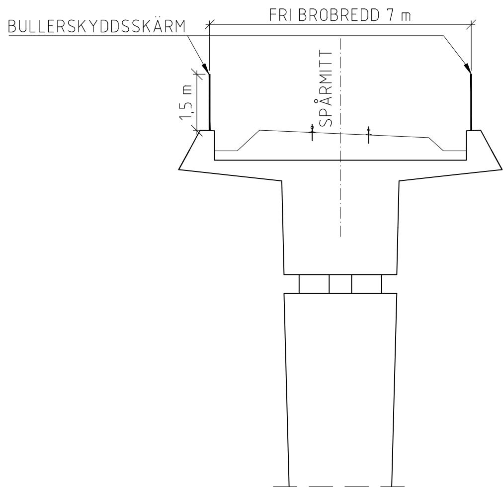
SEKTION B-B SKALA 1:100
