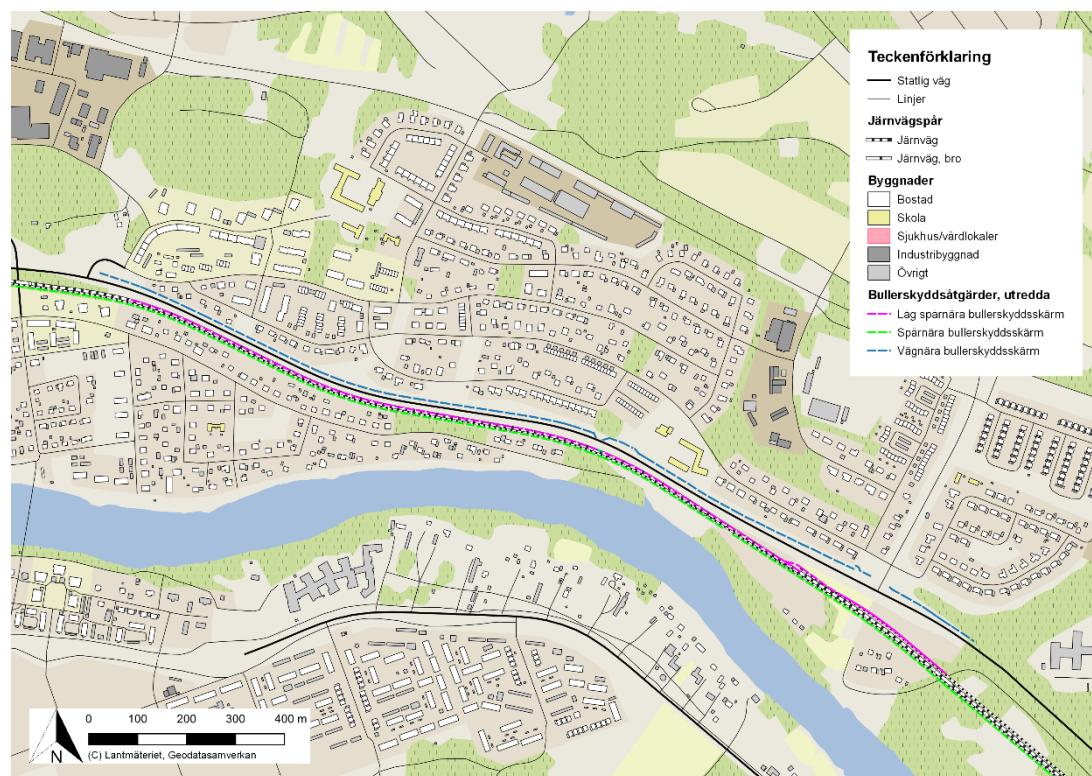
Figur 6.4: Utredda bullerskyddsåtgärder i område 2: Hedensbyn - Morön.
