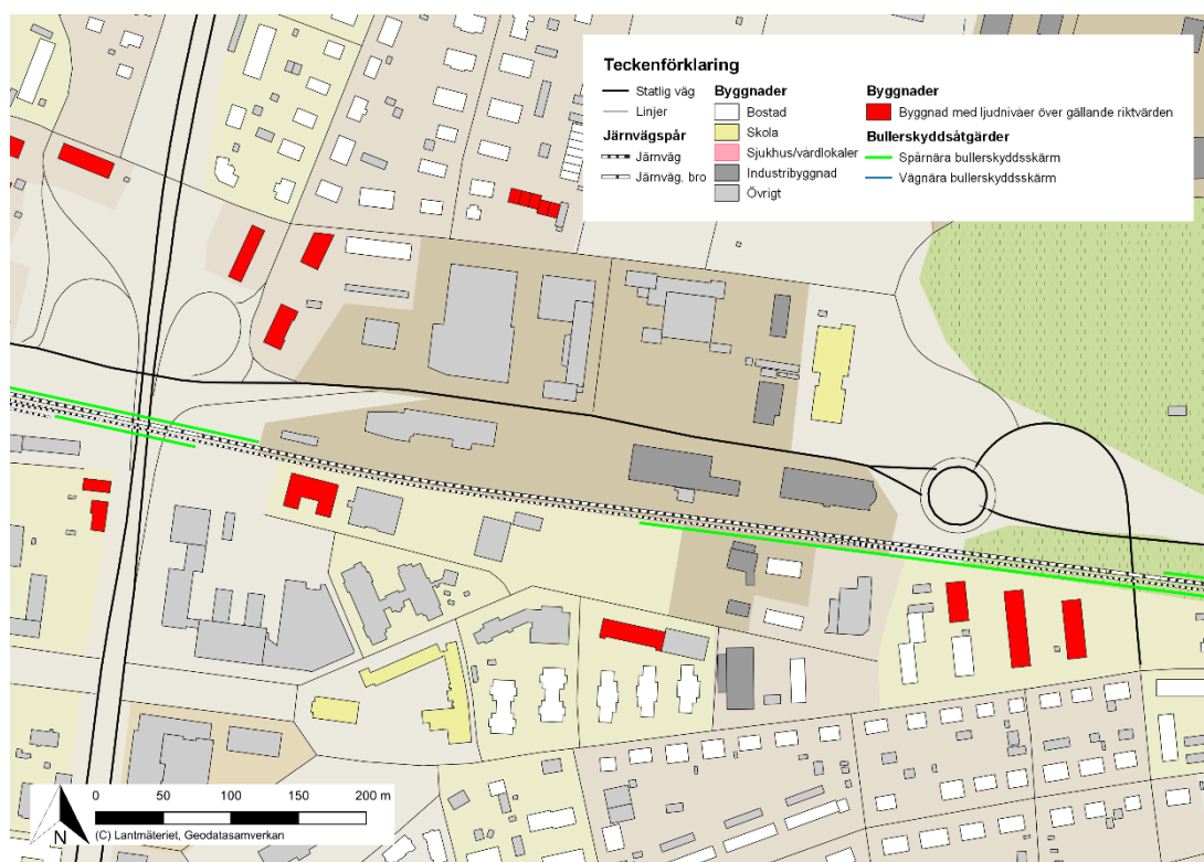
Figur 6.11: Byggnader med ljudnivåer över gällande riktvärden med spår- och vägnära bullerskyddsåtgärder.
