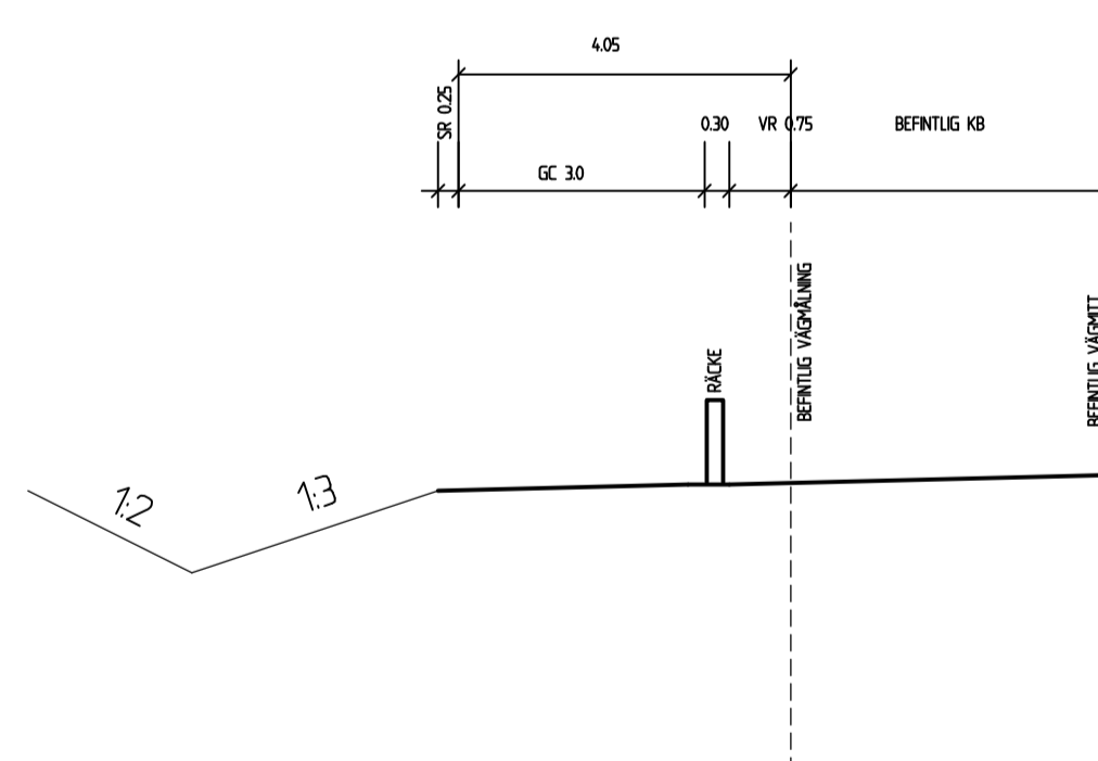
BREDDNING AV VÄG 600 FÖR GC-VÄG
