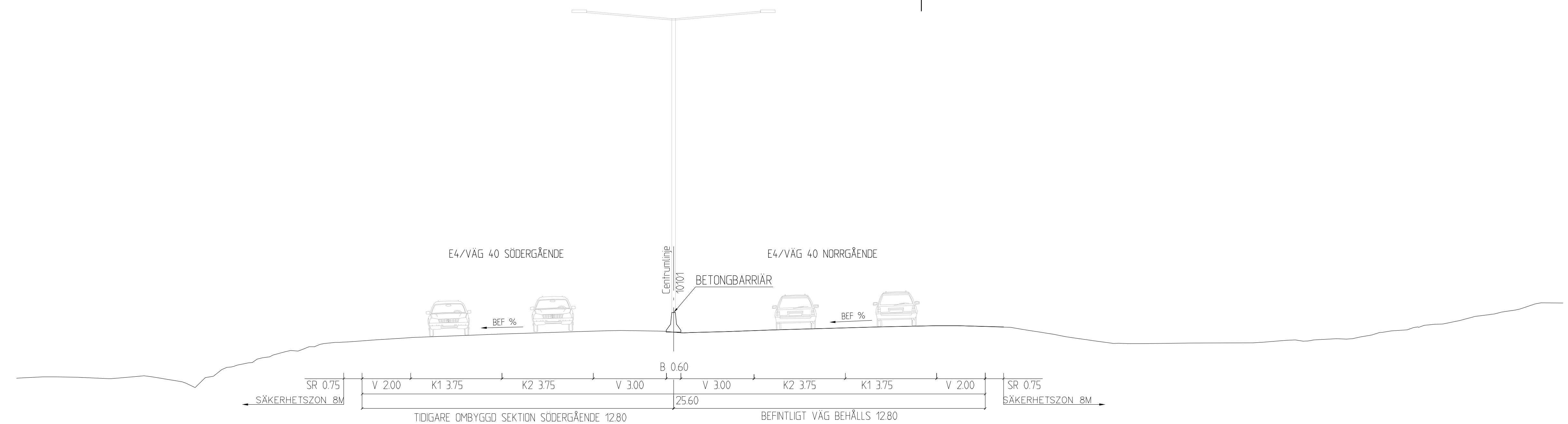
TYPSEKTION 07 E4 (MITTFÖR TRAFIKPLATS RYHOV) VÄGLINJE 10101, 3/250
