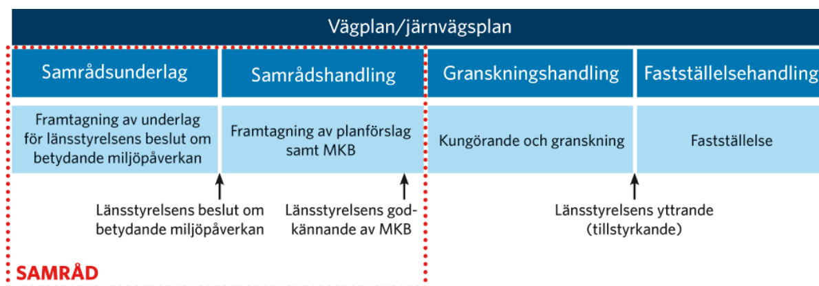
Figur 4. Trafikverkets planläggningsprocess.
