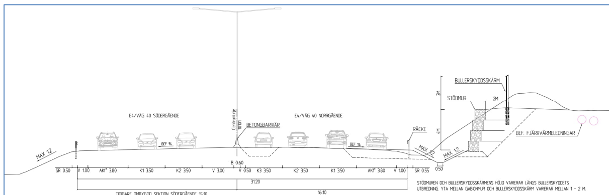
Figur 31. Typsektion för delen förbi bostadsområdet Ljungarum.
