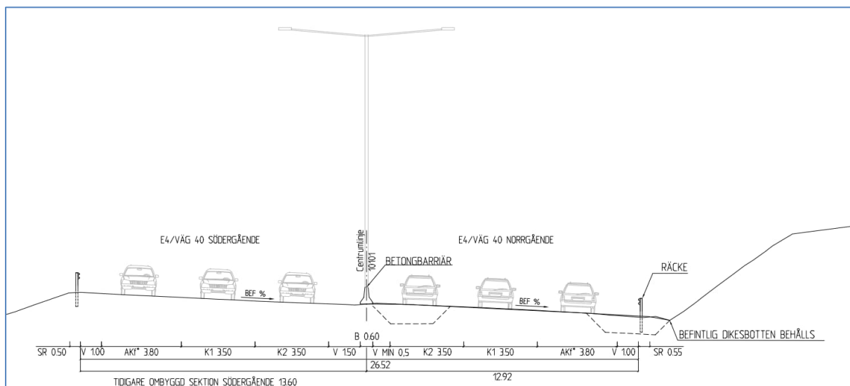
Figur 32. Typsektion för delen förbi Ryhovs herrgård.
