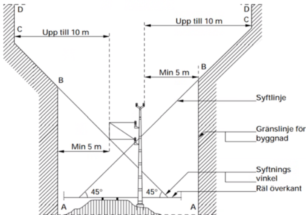
Figur 22. Säkerhetsavstånd för byggnader. Källa ELSÄK-FS 2008:1.
