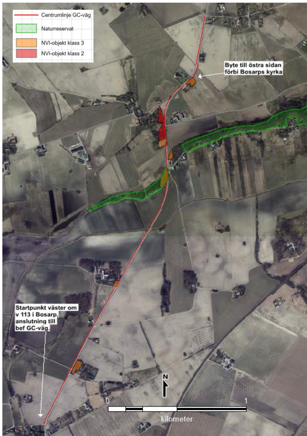
Figur 28. Planskiss över alternativ 1, med gång- och cykelväg huvudsakligen förlagd väster om väg 113.
