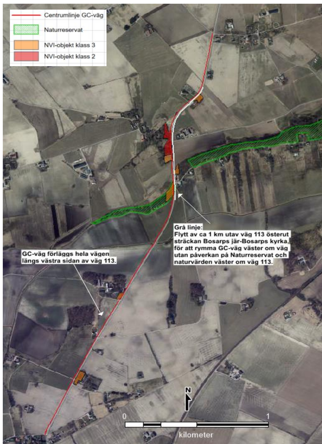
Figur 29. Planskiss över alternativ 2. Längs vitmarkerad sträcka flyttas väg 113 österut, för att gång- och cykelväg ska rymmas väster om väg 113, utan intrång i Bosarps jär och naturvärden väster om väg 113.
