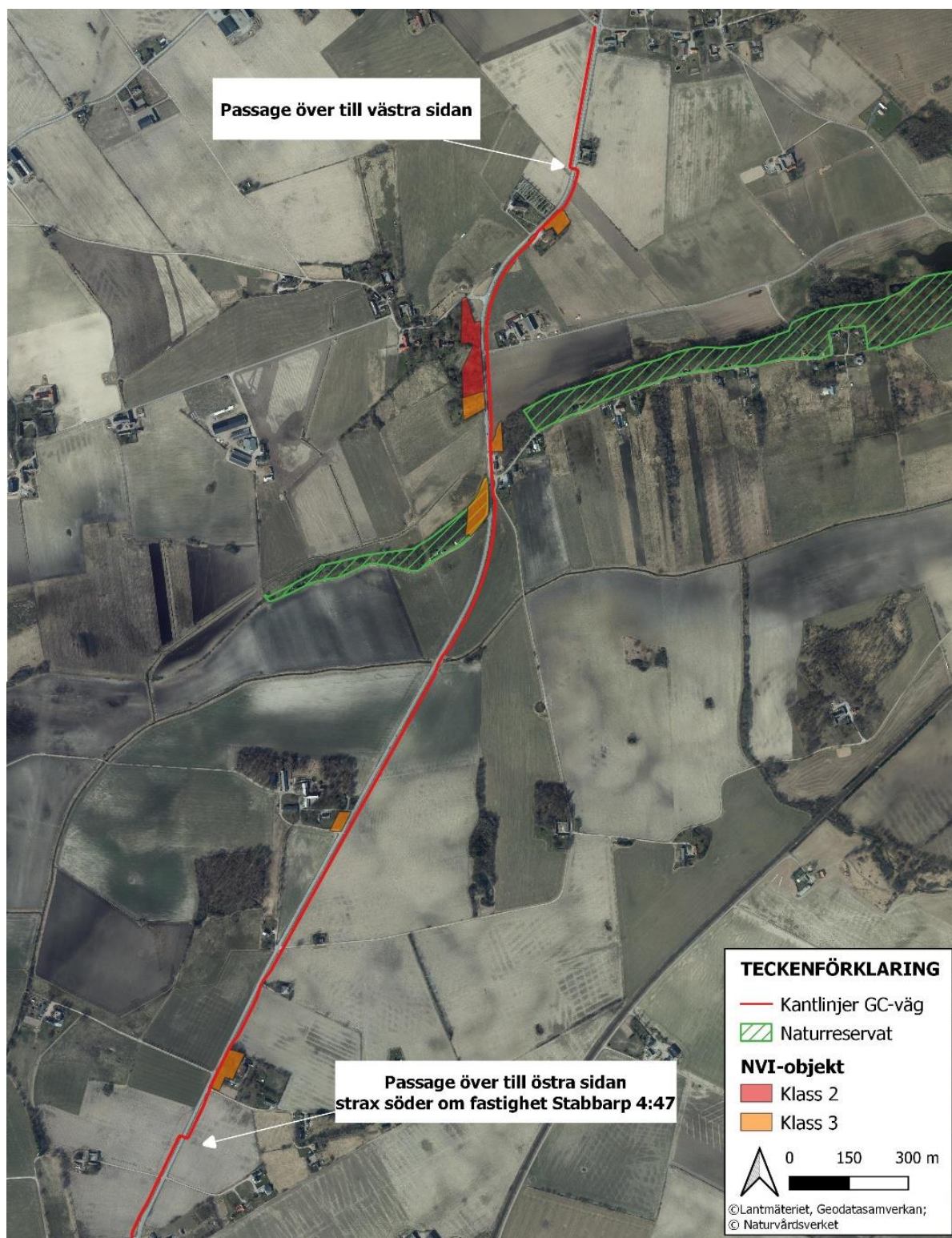
Figur 26. Planskiss över föreslagen sträckning. Gång- och cykelvägen är förlagd till viss del öster om väg 113, för att undvika påverkan på Bosarps jär och naturvärden väster om väg 113.
