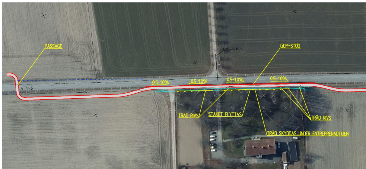
Figur 40. Planerad gång- och cykelväg och inmätta träd som ska rivas i södra delen av sträckan, vid Stabbarpsgården. Ortofoto © Lantmäteriet, Geodatasamverkan.
