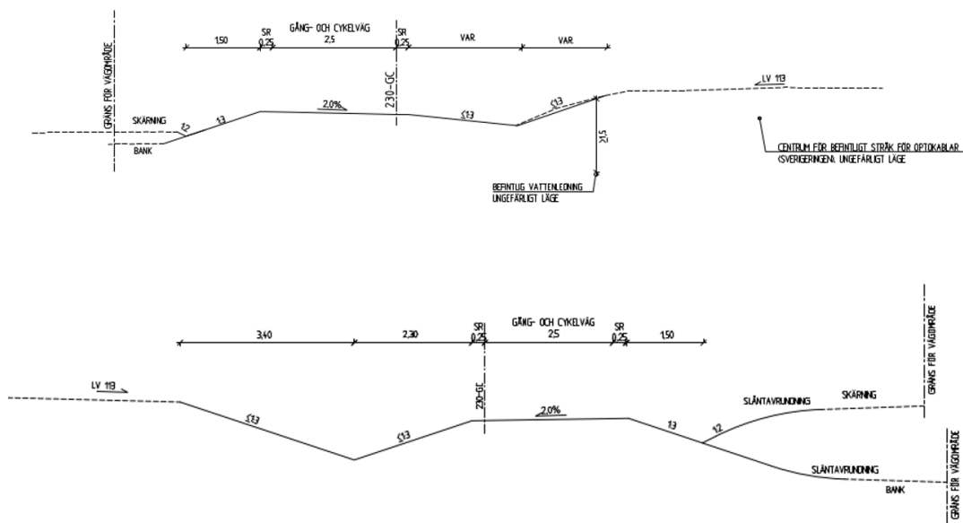
Figur 31. Typsektion D2.
