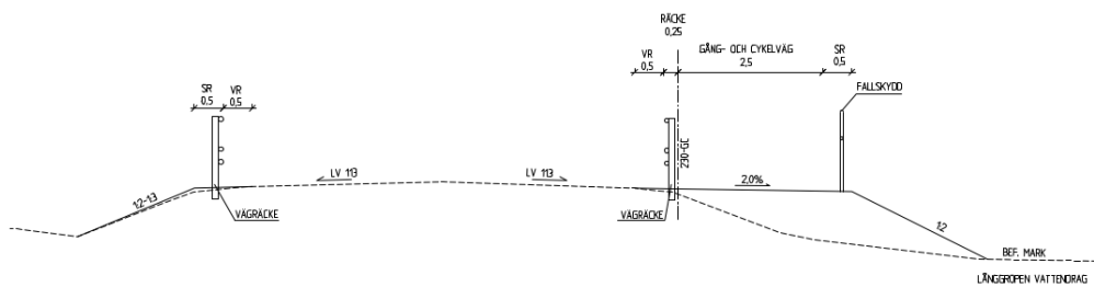
Figur 32. Typsektion F förbi Långgropen
