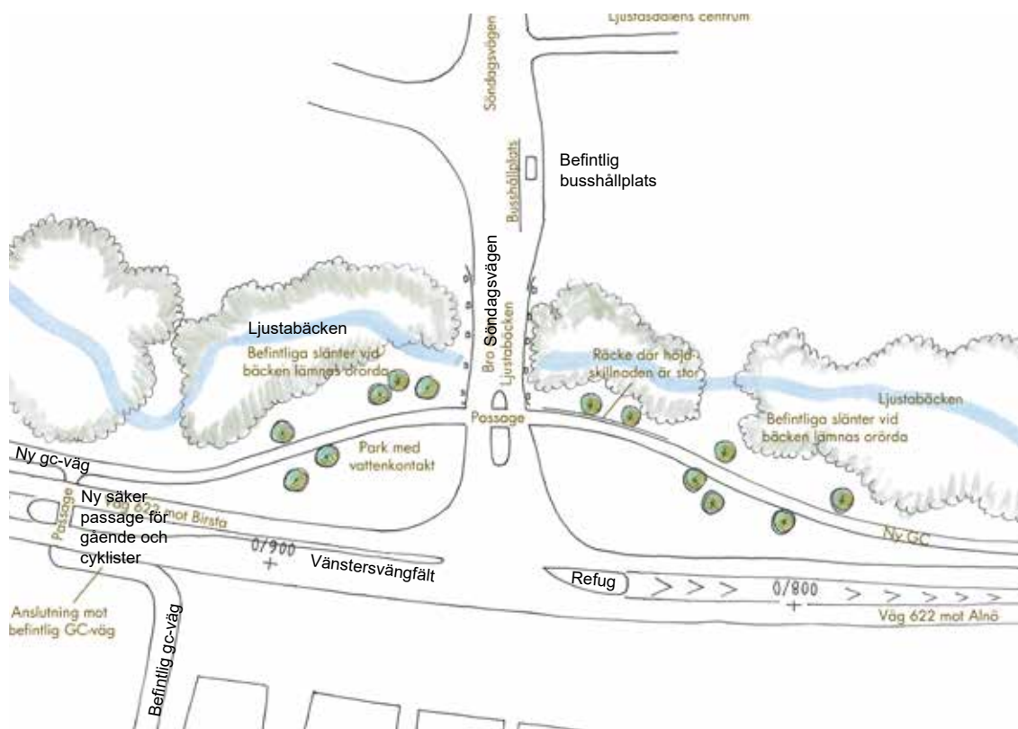
Figur 5.6 Illustration visande korsningen med Söndagsvägen. Gång- och cykelvägen följer Ljustabäcken och svänger in mot centrumbebyggelsen i Ljustadalen. Avståndet mellan gång- och cykelvägen och väg 622 behövs för trafiksäkerheten i korsningen. En parkliknande yta skapas som dessutom ger en mer vilksam miljö för de gående.
