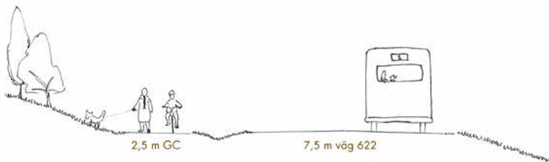
Figur 5.1 Illustration visande hur väg och gångväg förhåller sig till varandra där gång- och cykelvägen ligger separerat från väg 622. De separeras av ett flackt dike sått med gräs. Dikets bredd är 3 meter.
