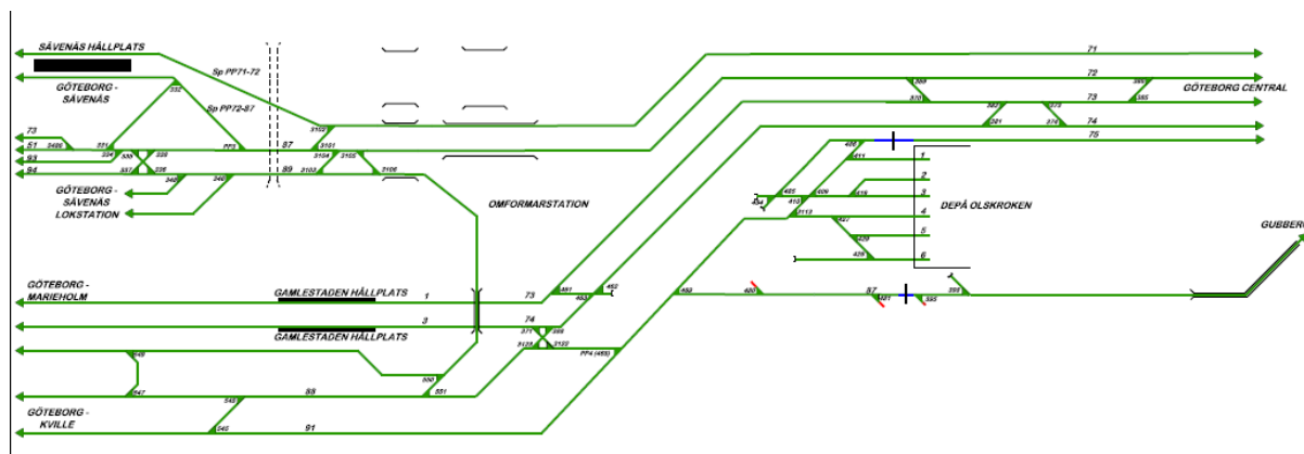
Figur 6 Spårplan Olskroken 2021-10-11 -- 2022-07-24
