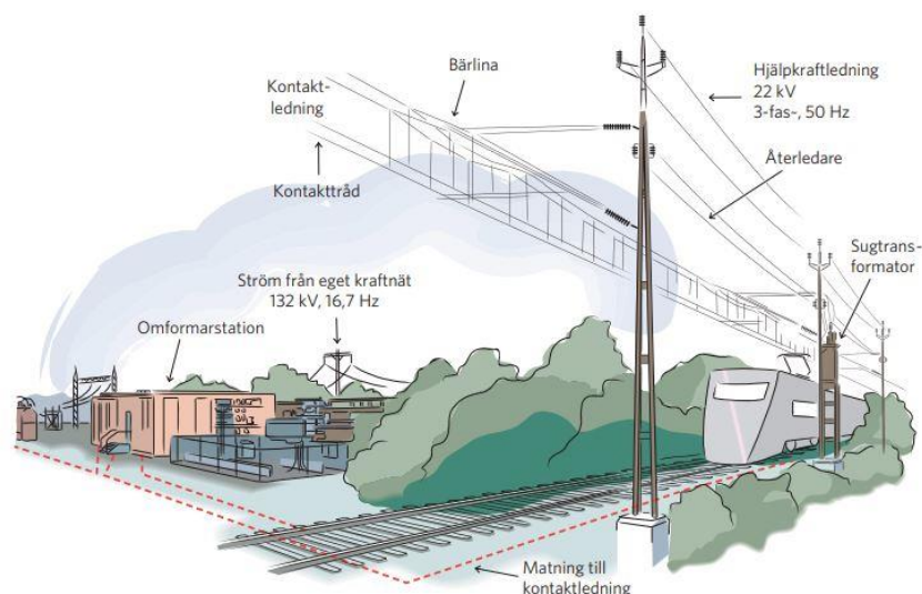
Figur 5.1-1. Järnvägens elanläggning.
