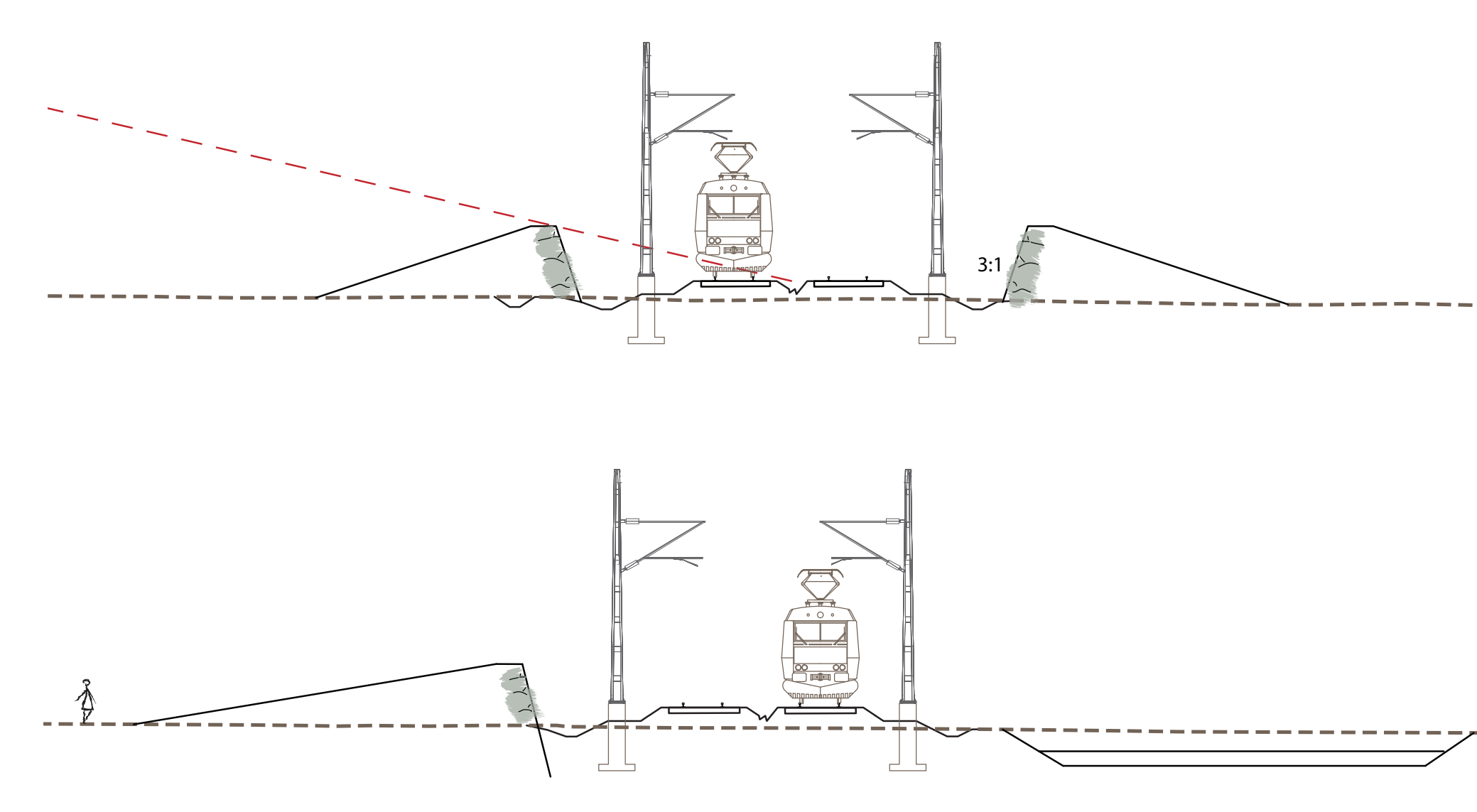
Schematiska principskisser över möjlig utformning av bullerskyddsåtgärder söder om tunnelmynningen.
