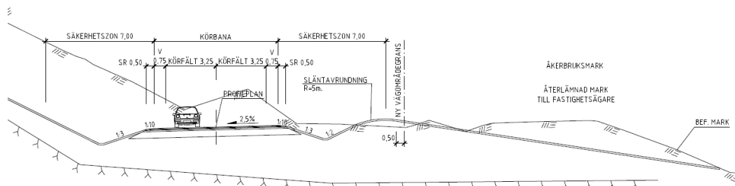
Figur 5.2-9. Sektion mellan 29/300 och 29/500. På högra sidan av vägen visas hur marken återställs.
