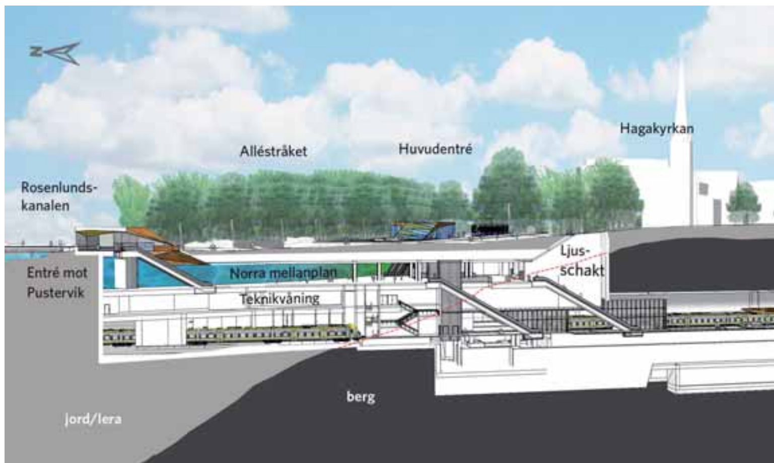
FIGUR 6.7. Sprängskiss genom stationen
