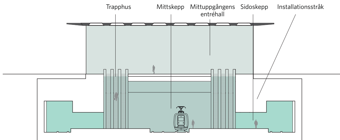
FIGUR 5.13. Tvärsektion med midskeppet och sidoskeppen tagen vid mittuppgången. Man ser tydligt skillnaden i rumslighet. Taket i midskeppet reser sig mot uppgången och bildar stationsrummets högsta punkt. Under installationsstråken sänks takhöjden och bildar sidoskeppens intimare rum.
