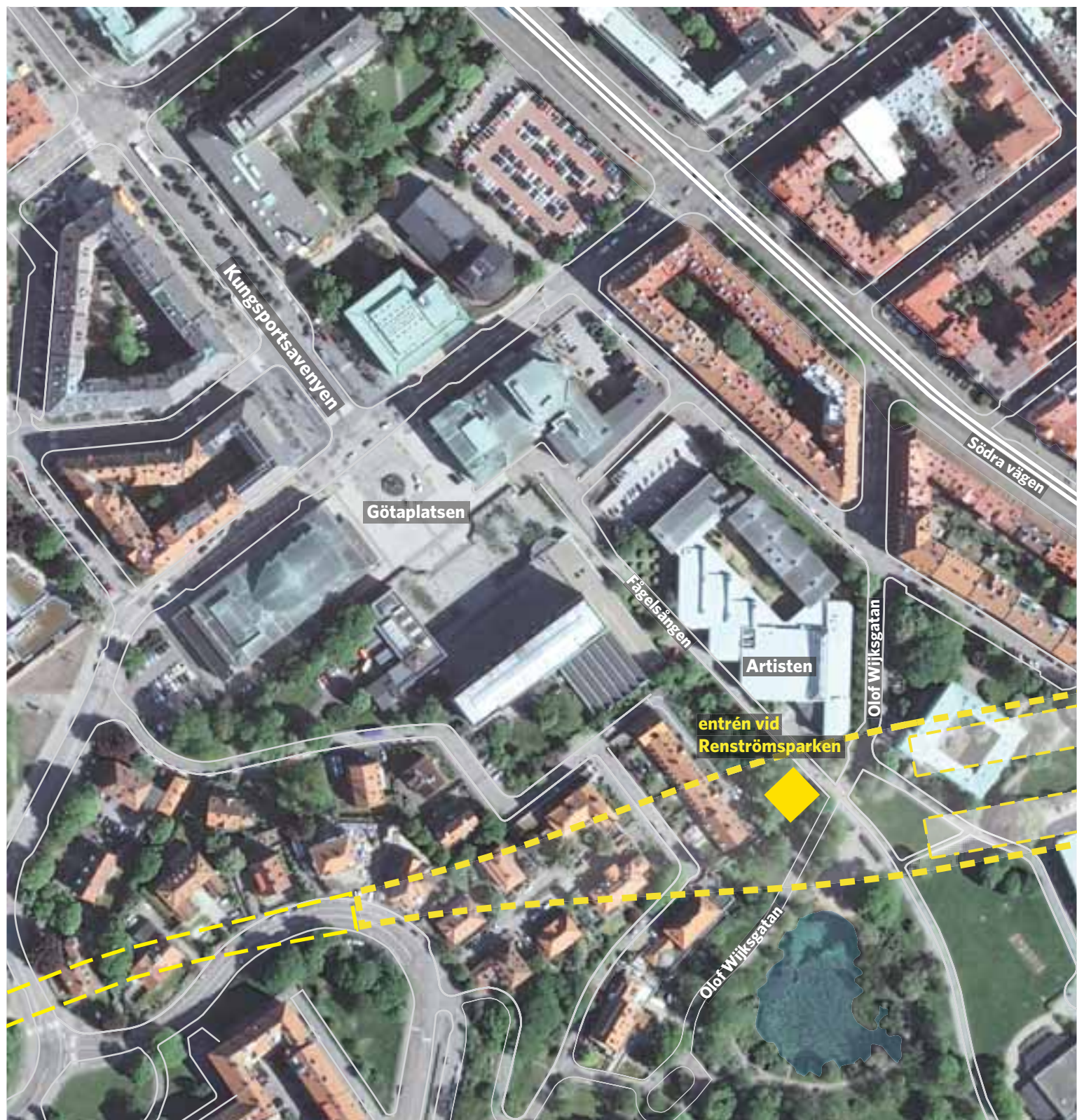
FIGUR 7.2. Situationsplan som visar stationens läge och placering av entréerna.
