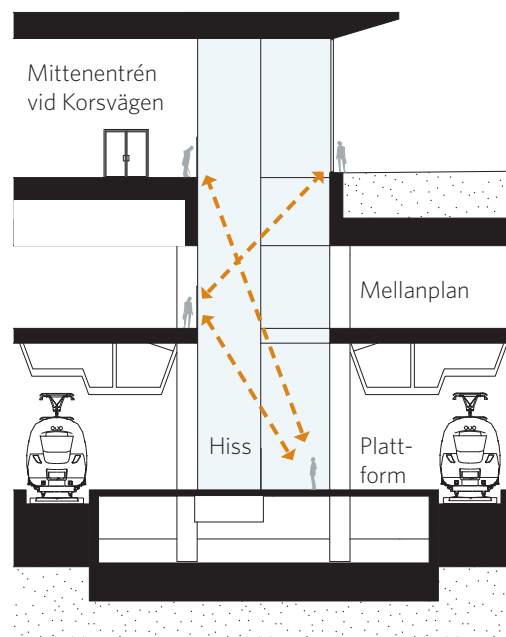
FIGUR 7.33. Bilden visar den visuella kontakten mellan våningsplanen vid Korsvägens mittenentré. Hissarna kan här gå från plattform och hela vägen upp till entrén.
