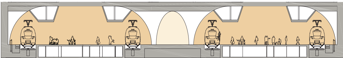
FIGUR 7.29. Tvärsektion genom betongdelen med pelarfri plattform och valvformad betongkonstruktion vid ytterväggar och i mitten.
