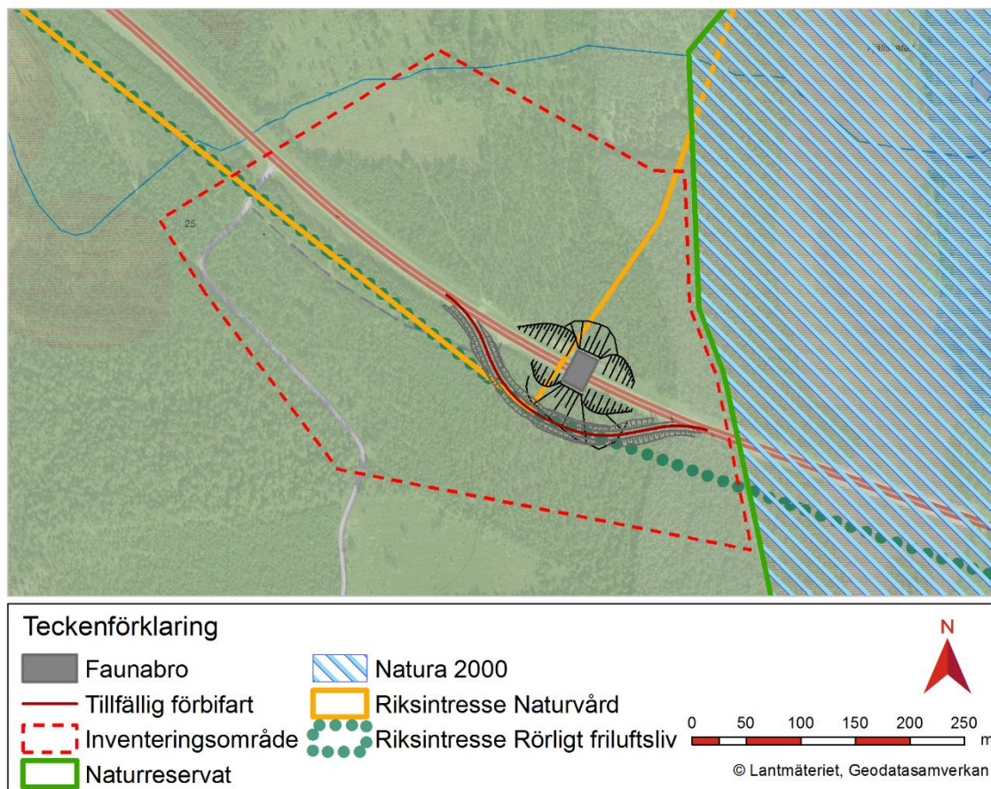
Figur 21. Planerad faunapassage och tillfällig förbifart under byggtiden.
