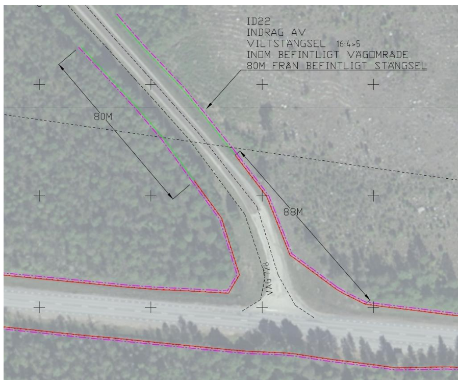
Figur 19. Illustration som visar hur indragning av stängsel vid allmän eller enskild väg med frekvent trafik kan utföras, utdrag från illustrationskarta.
