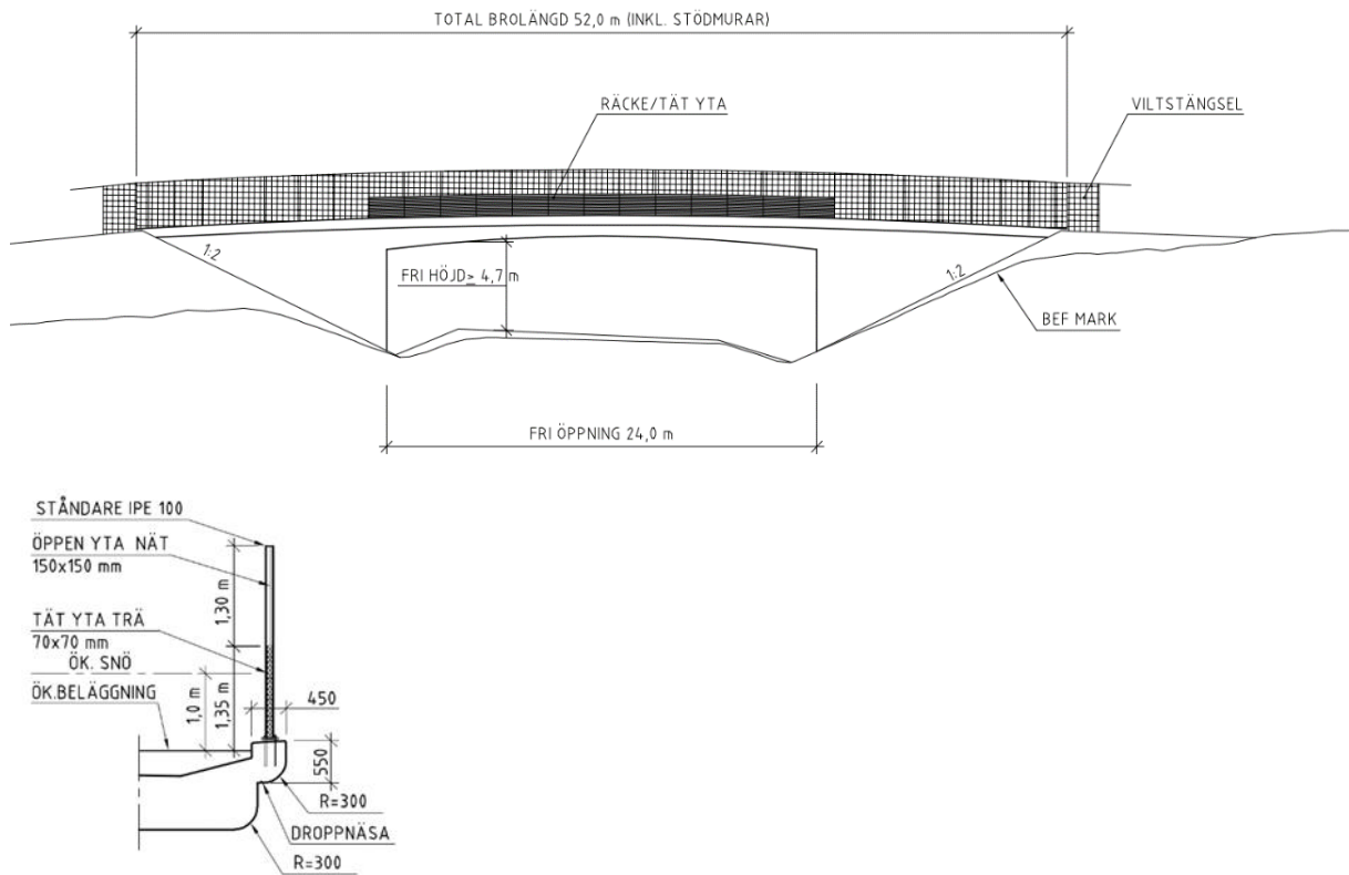
Figur 16. Vald brotyp – plattrambro, samt förslag till räckesutformning (principfigur).
