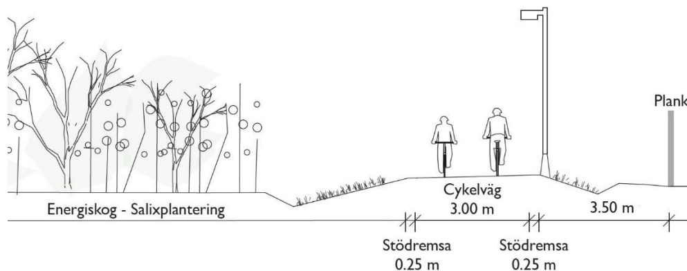
Figur 34 Principskiss för Bergströmshusen
