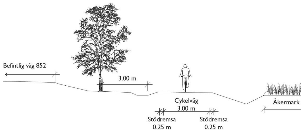
Figur 32 Principskiss för Kyrkstigen – Stora Uppåkravägen
