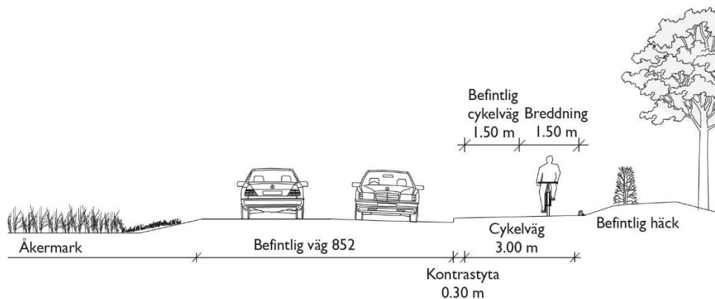
Figur 30 Principskiss för Vallgården, norra delen
