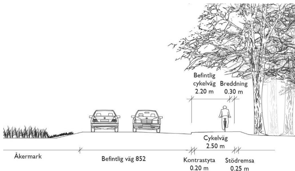
Figur 29 Principskiss för Vallgården, södra delen
