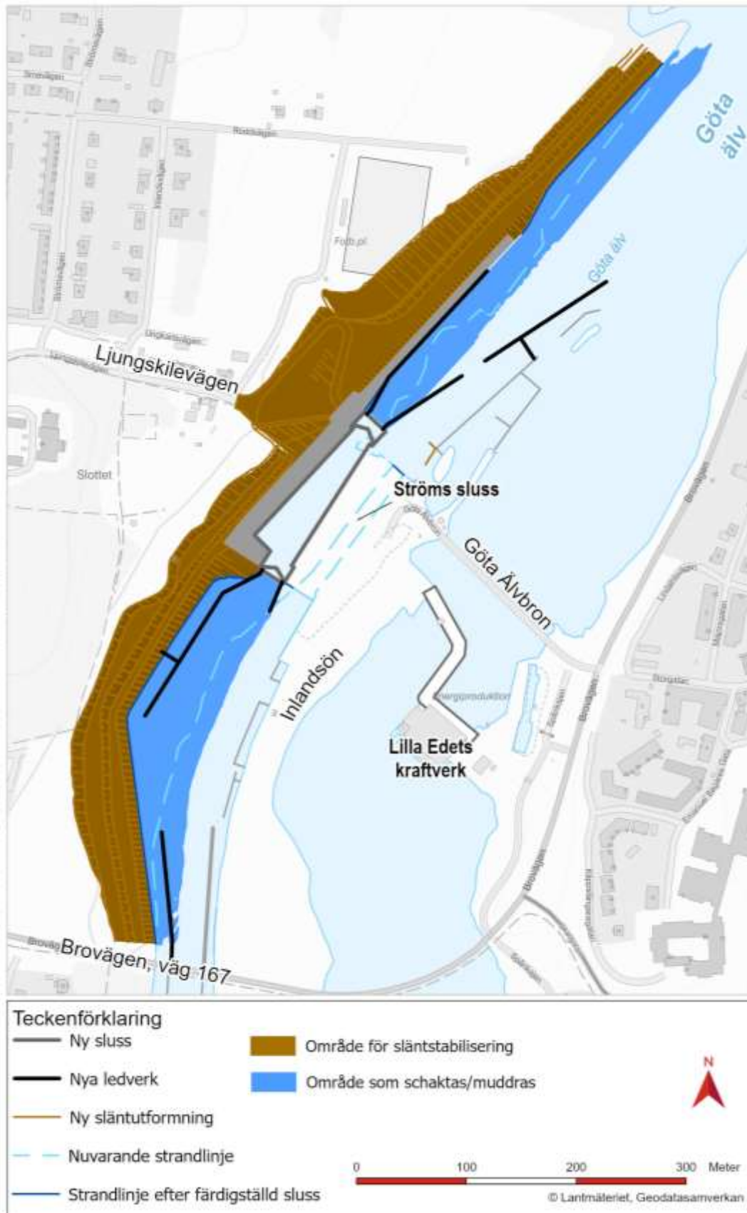
Figur 11. Ungefärligt område för ny släntutformning- och stabilisering samt muddring vid ny sluss, nya ledverk och anpassning av farled.
