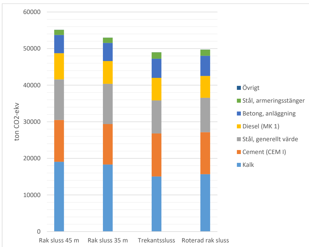
Figur 27. Bedömd klimatpåverkan från byggskedet för de fyra slussalternativen, fördelat enligt bidrag från olika material och arbetsmoment.
