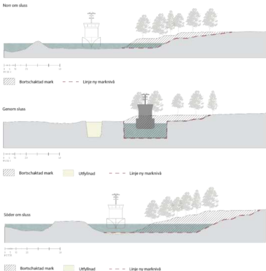
Figur 18. Principskisser på typsektioner vid olika delar av slussleden.
