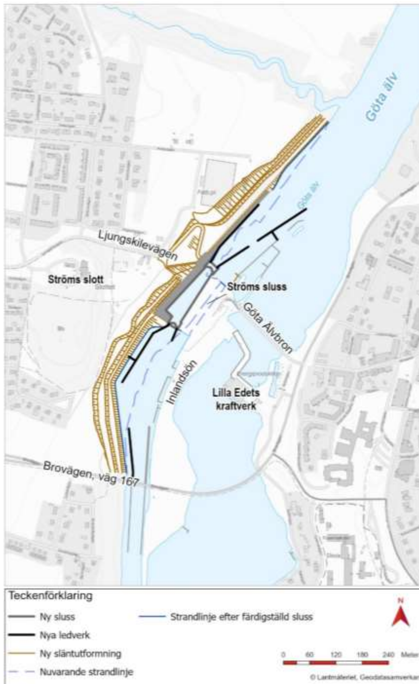
Figur 6. Ny slussanläggning och ny släntutformning.
