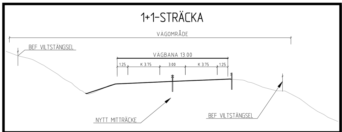
Figur 16. Typsektion 1+1
