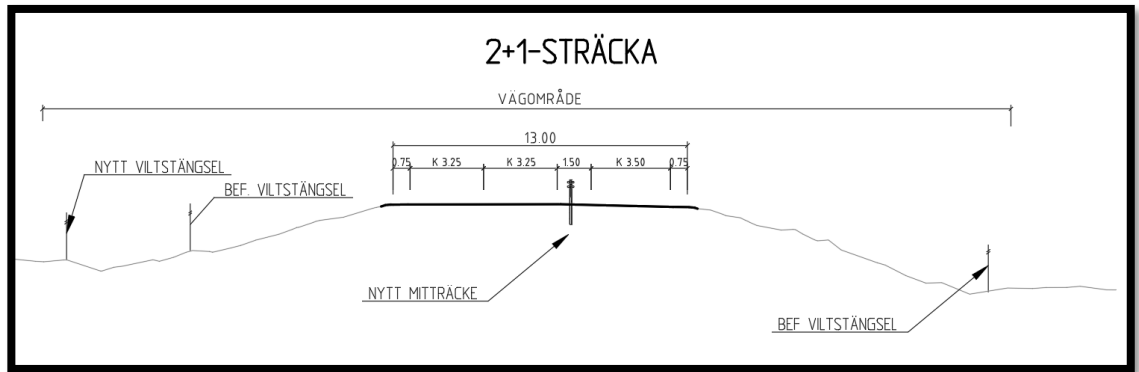
Figur 15. Typsektion 2+1
