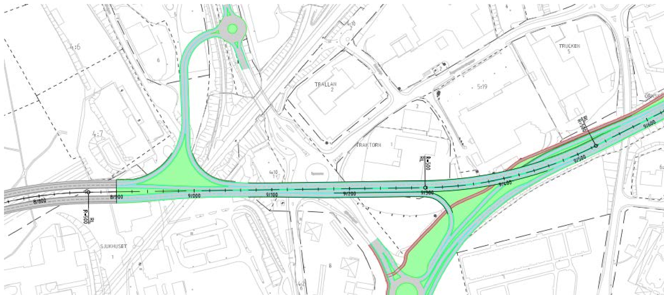
Alternativ 1 Norra trafikplatsen variant med 500 m radie – Bilaga 4
