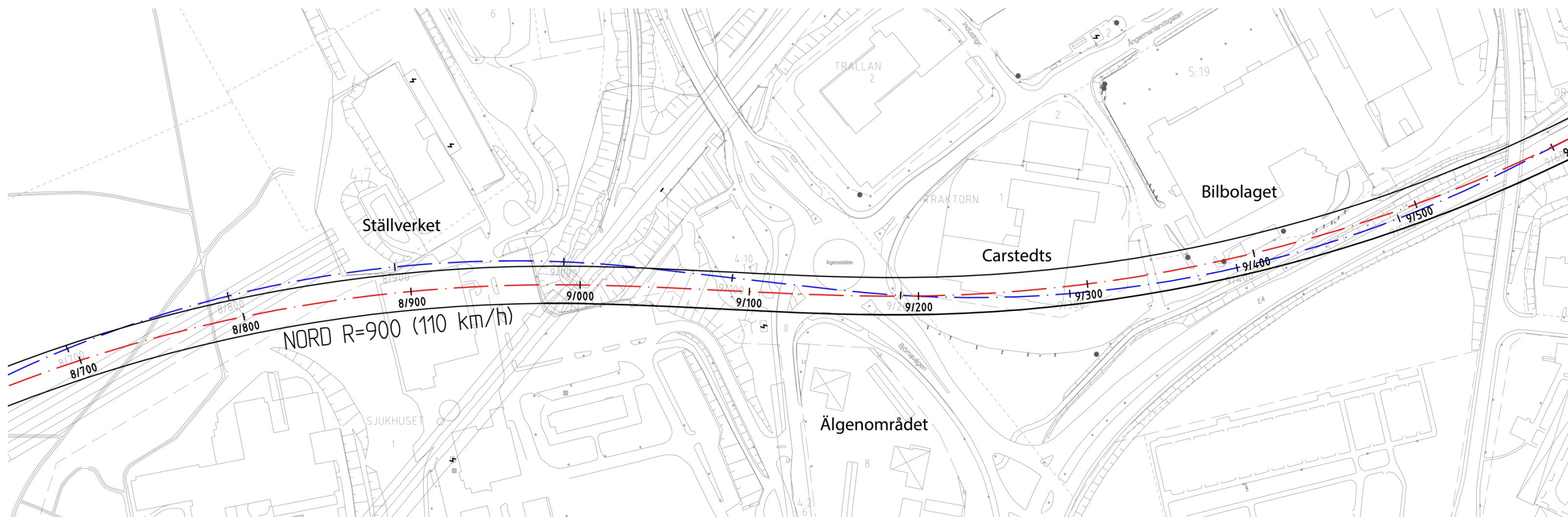
Alternativ 1 Norra trafikplatsen variant med 900 m radie – Bilaga 5
