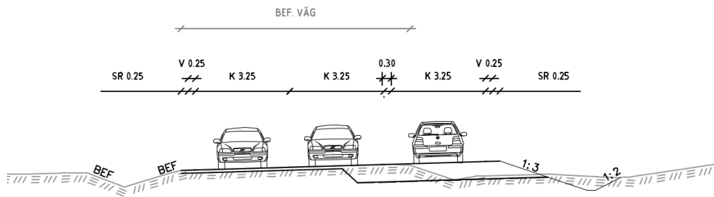
Figur 15. Fokusområde 1, sektion.
