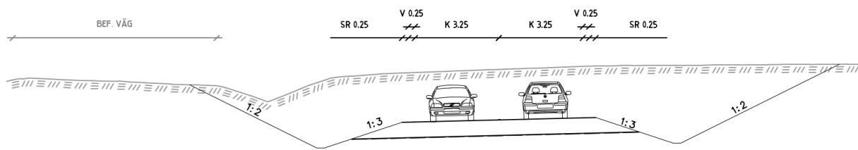
Figur 17. Fokusområde 2, sektion.
