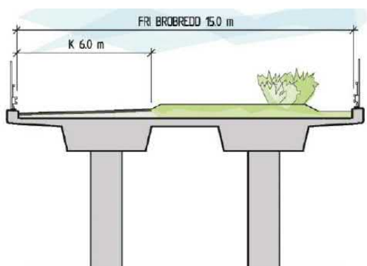
Figur 4.2.19. Sektion A-A för faunaanpassad vägbro över E20 vid Motorp.
