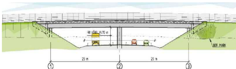
Figur 4.2.18. Faunaanpassad vägbro över E20 vid Motorp.
